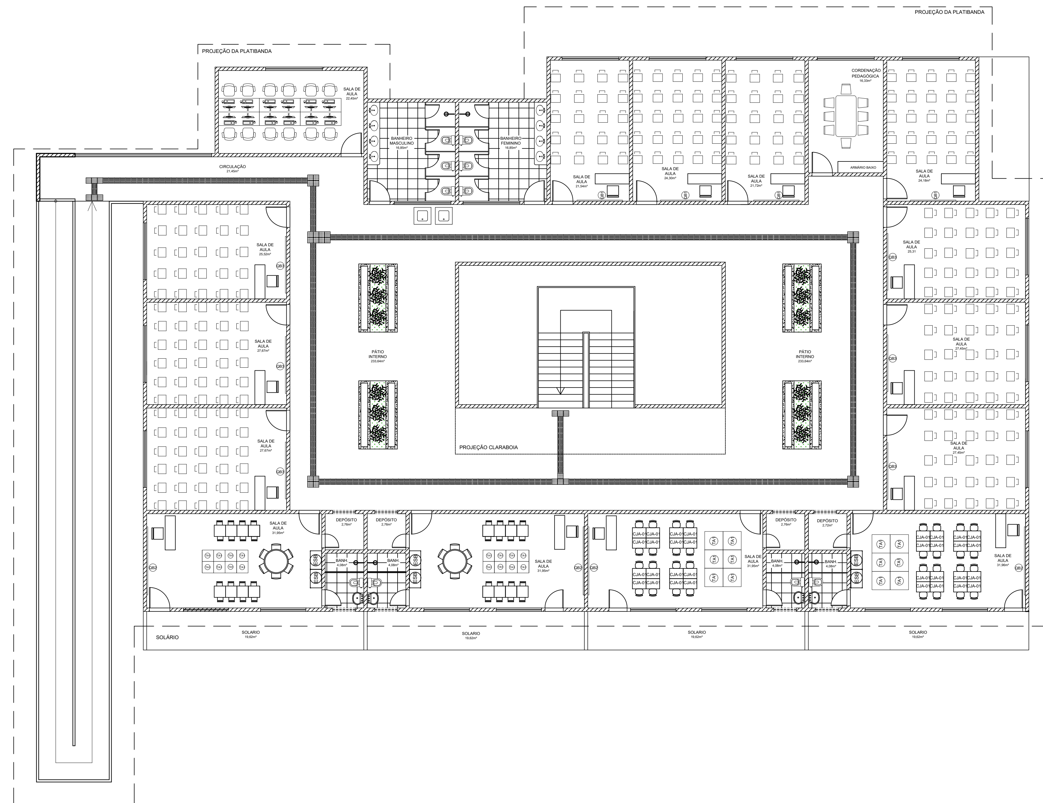
1 PLANTA LAYOUT 2° PAVIMENTO ESCALA 1/100
