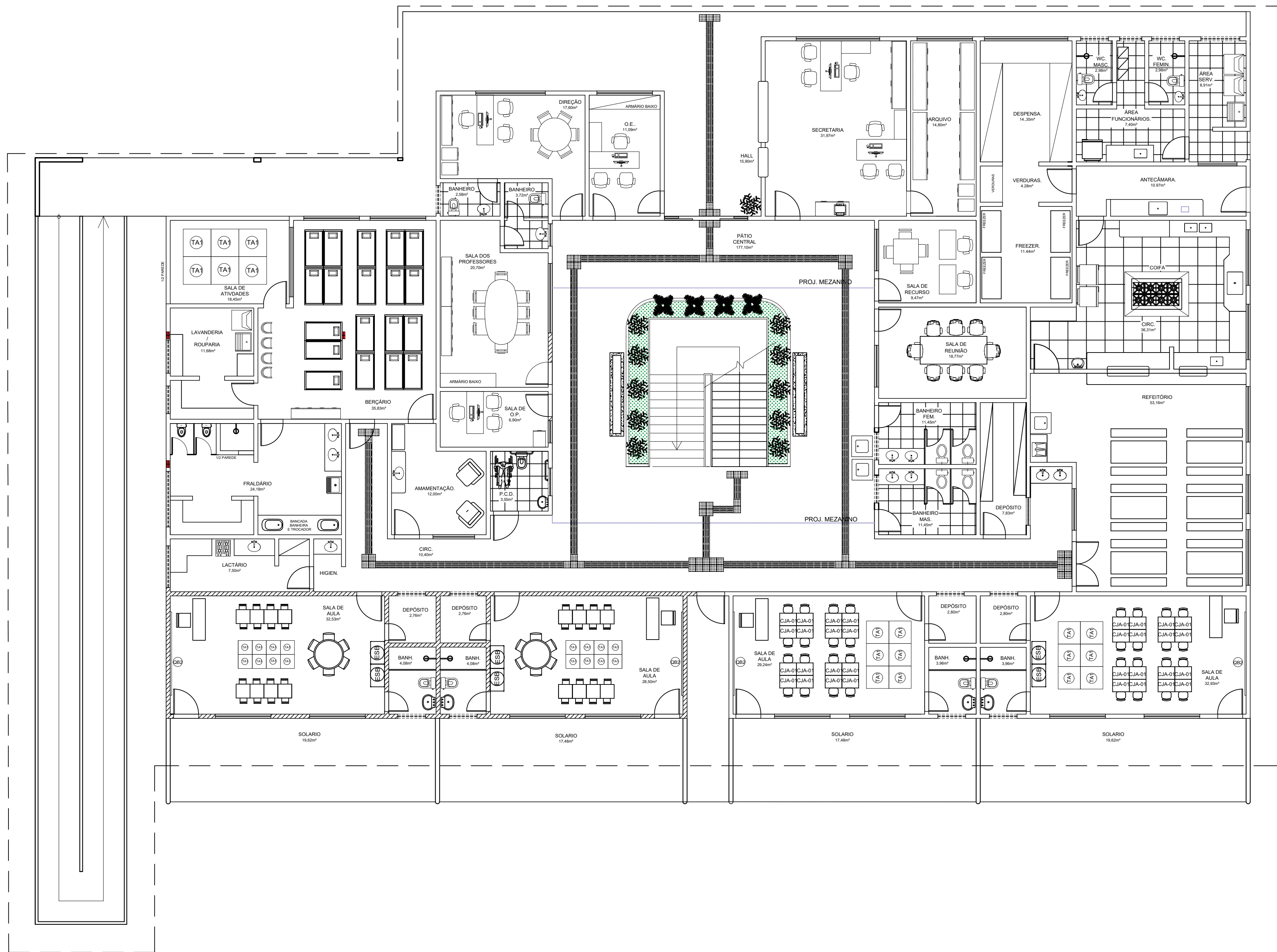
1 PLANTA LAYOUT 1° PAVIMENTO ESCALA 1/100
