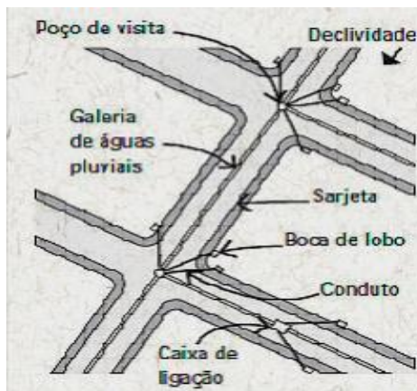
Figura 3: Sistema de rede de drenagem
