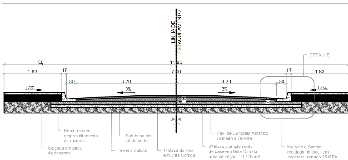
Figura 1 - Seção Tipo pavimento
