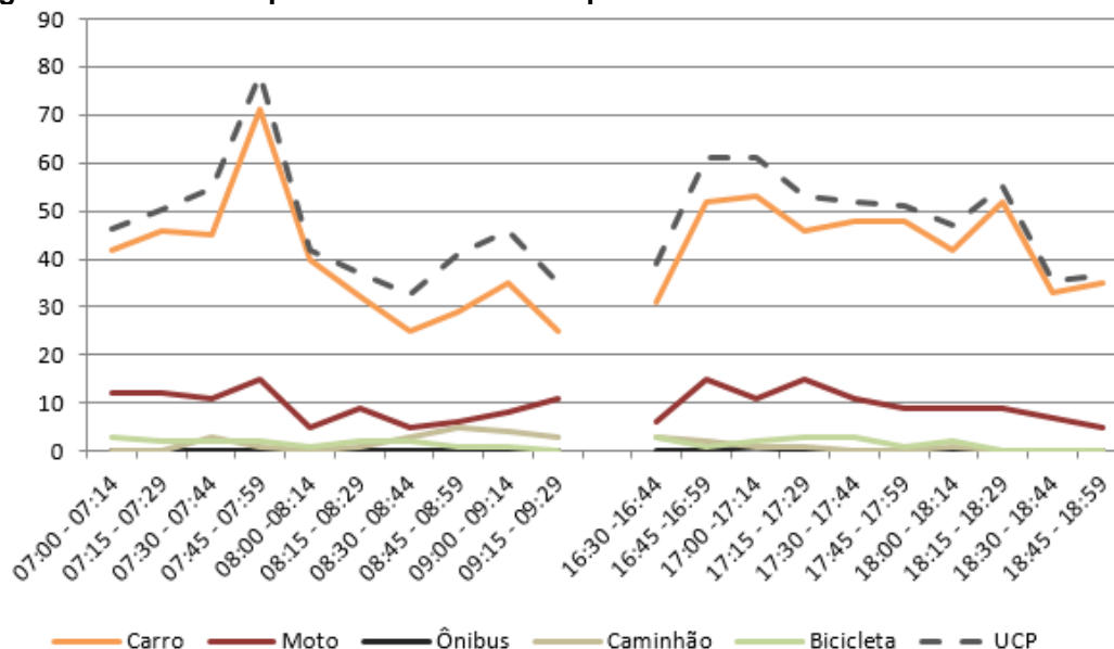
Figura 241 – Gráfico quantidade de veículos para cada intervalo de 15 minutos no M 7
