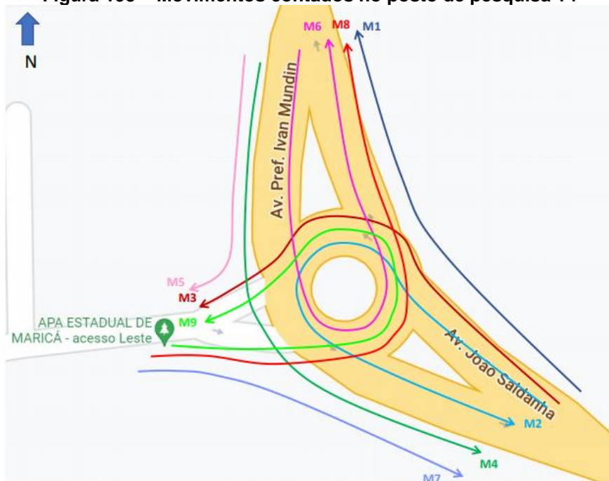
Figura 198 – Movimentos contados no posto de pesquisa 14
