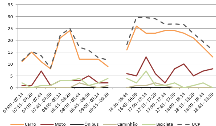
Figura 91 – Gráfico quantidade de veículos para cada intervalo de 15 minutos no M 10
