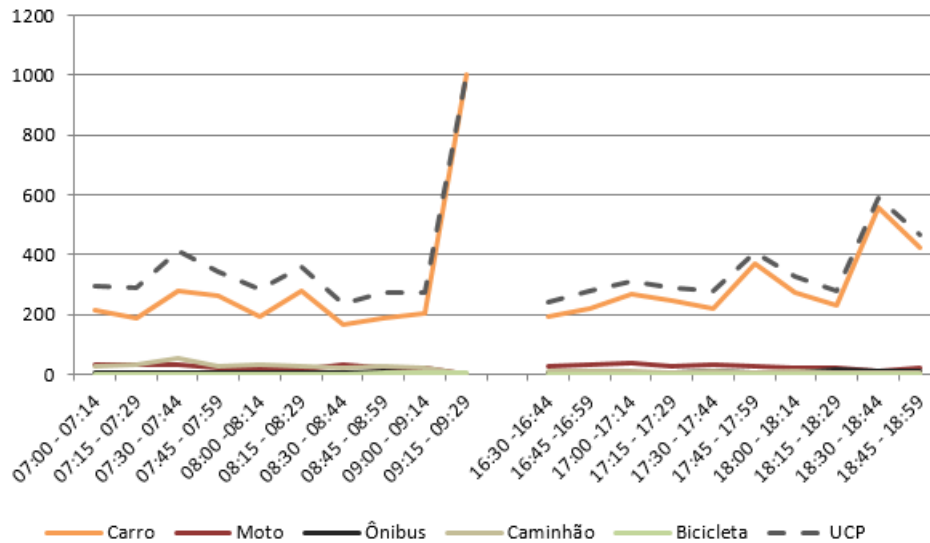
Figura 70 – Gráfico quantidade de veículos para cada intervalo de 15 minutos no M 2
