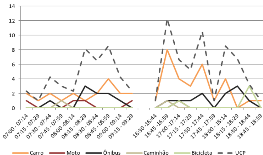
Figura 148 – Gráfico quantidade de veículos para cada intervalo de 15 minutos no M 1
