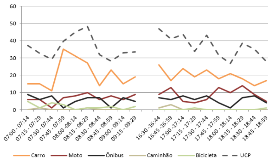
Figura 250 – Gráfico quantidade de veículos para cada intervalo de 15 minutos no M 2
