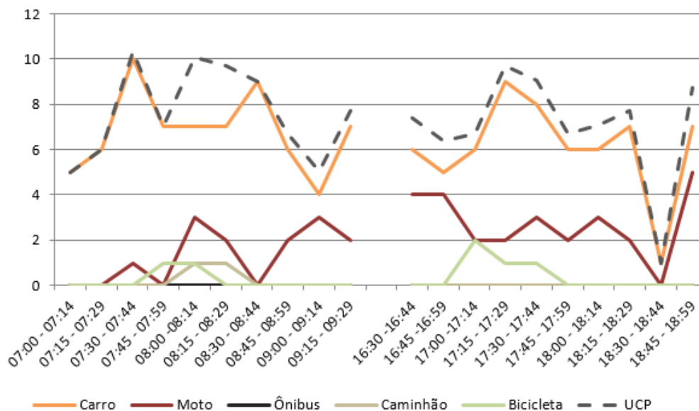
Figura 160 – Gráfico quantidade de veículos para cada intervalo de 15 minutos no M 13
