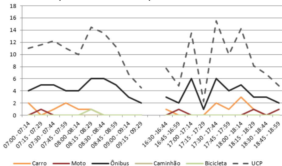
Figura 101 – Gráfico quantidade de veículos para cada intervalo de 15 minutos no M 6
