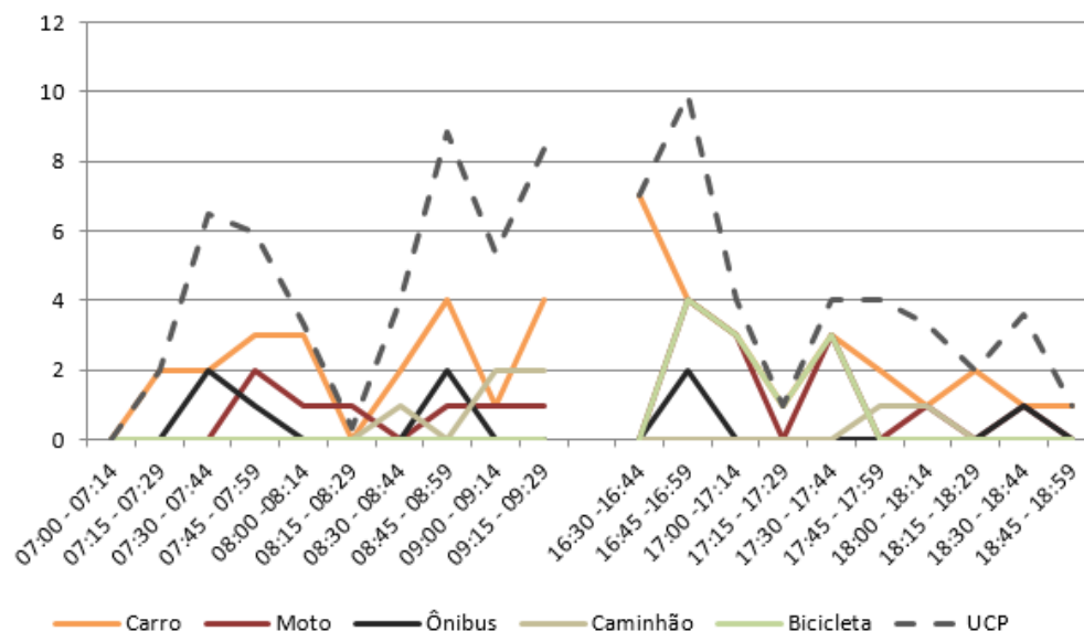
Figura 202 – Gráfico quantidade de veículos para cada intervalo de 15 minutos no M 3
