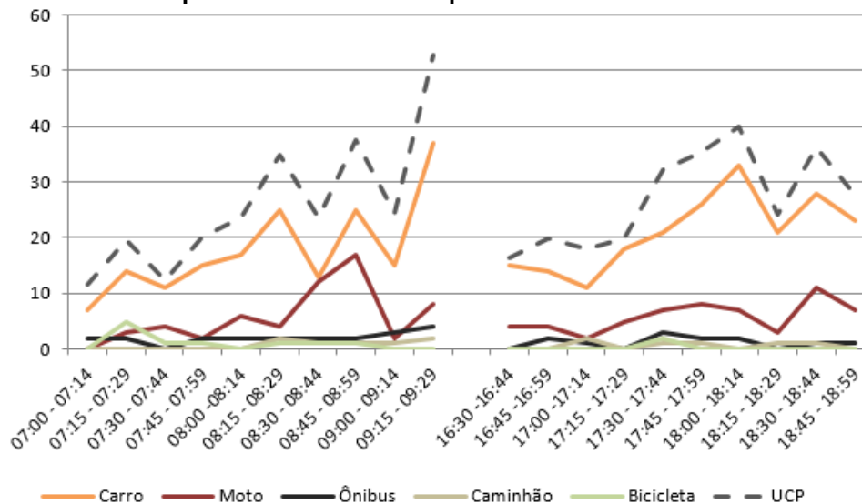
Figura 228 – Gráfico quantidade de veículos para cada intervalo de 15 minutos no M 12
