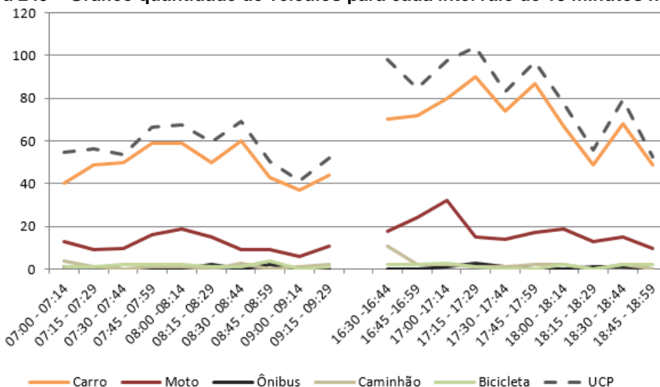
Figura 249 – Gráfico quantidade de veículos para cada intervalo de 15 minutos no M 1
