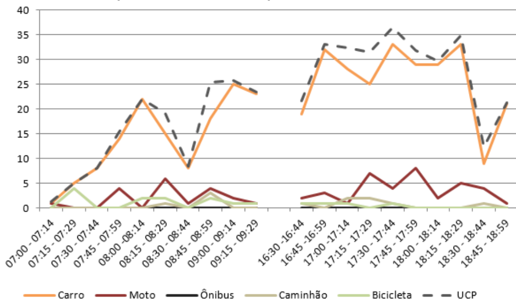
Figura 222 – Gráfico quantidade de veículos para cada intervalo de 15 minutos no M 6
