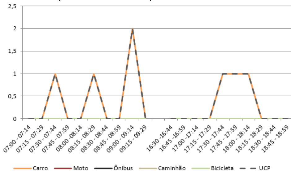
Figura 205 – Gráfico quantidade de veículos para cada intervalo de 15 minutos no M 6
