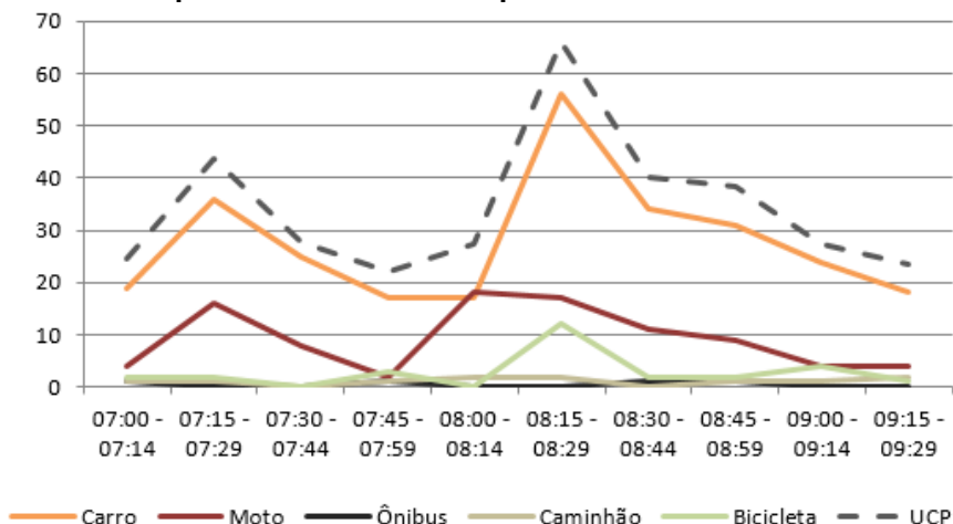
Figura 178 – Gráfico quantidade de veículos para cada intervalo de 15 minutos no M 11
