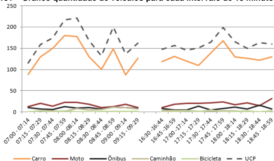
Figura 131 – Gráfico quantidade de veículos para cada intervalo de 15 minutos no M 5
