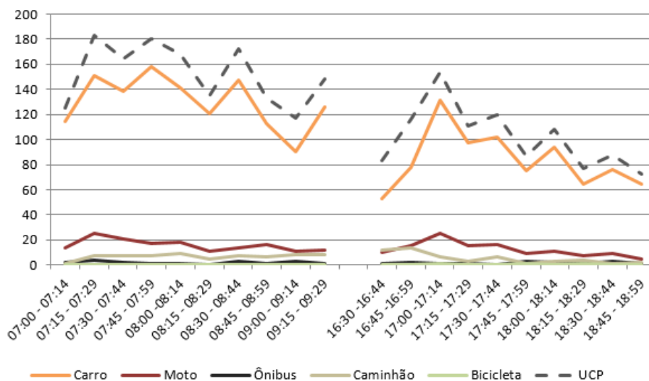
Figura 69 – Gráfico quantidade de veículos para cada intervalo de 15 minutos no M 1
