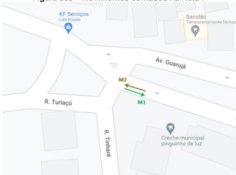
Figura 505 – Movimentos contados na Rota 7
