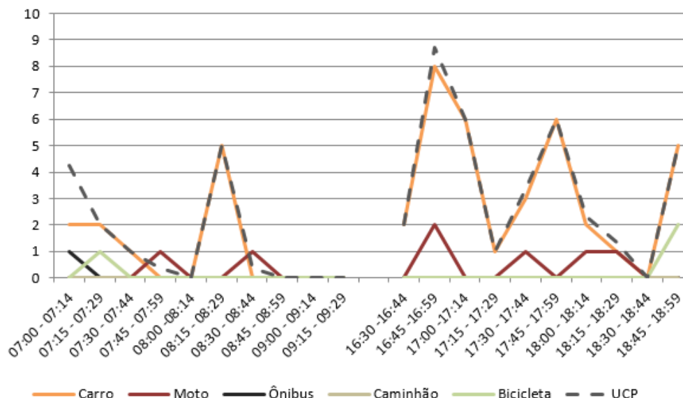
Figura 237 – Gráfico quantidade de veículos para cada intervalo de 15 minutos no M 3
