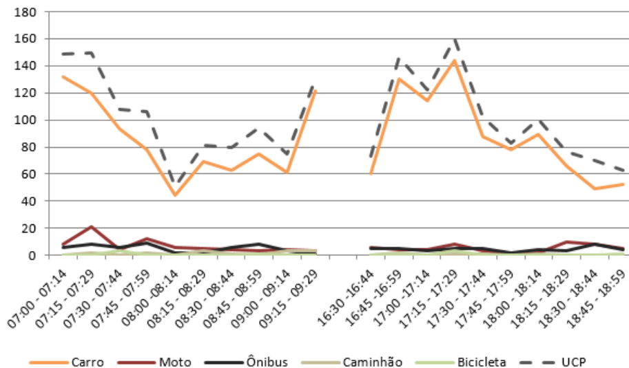
Figura 238 – Gráfico quantidade de veículos para cada intervalo de 15 minutos no M 4
