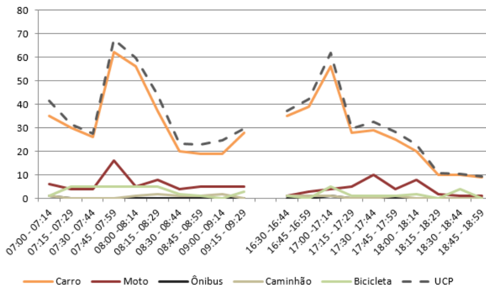
Figura 186 – Gráfico quantidade de veículos para cada intervalo de 15 minutos no M 2
