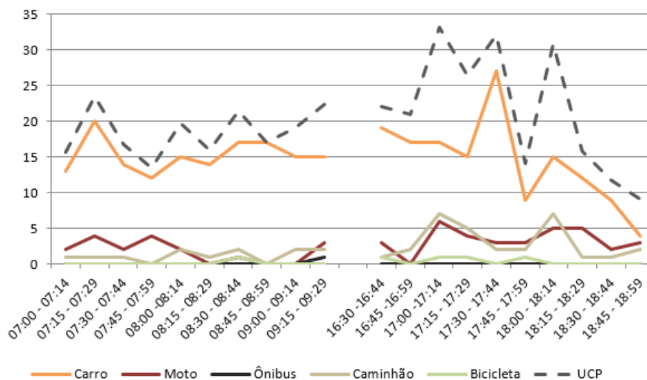
Figura 135 – Gráfico quantidade de veículos para cada intervalo de 15 minutos no M 9
