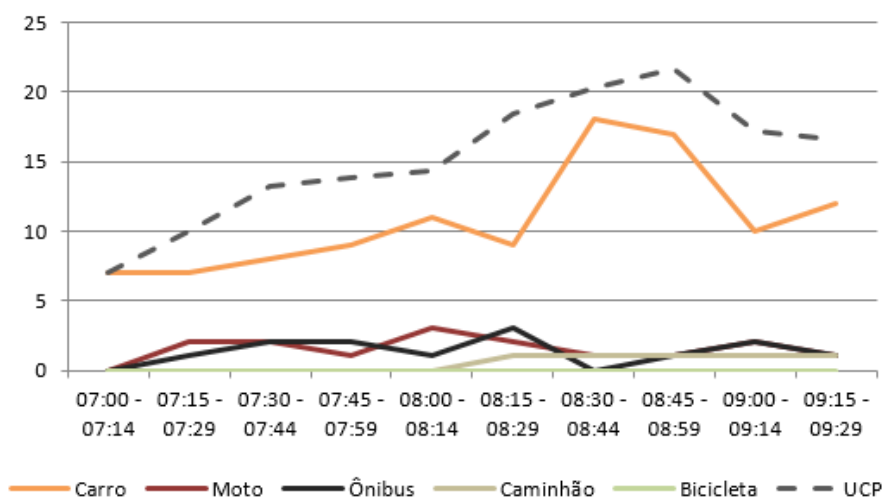
Figura 180 – Gráfico quantidade de veículos para cada intervalo de 15 minutos no M 13
