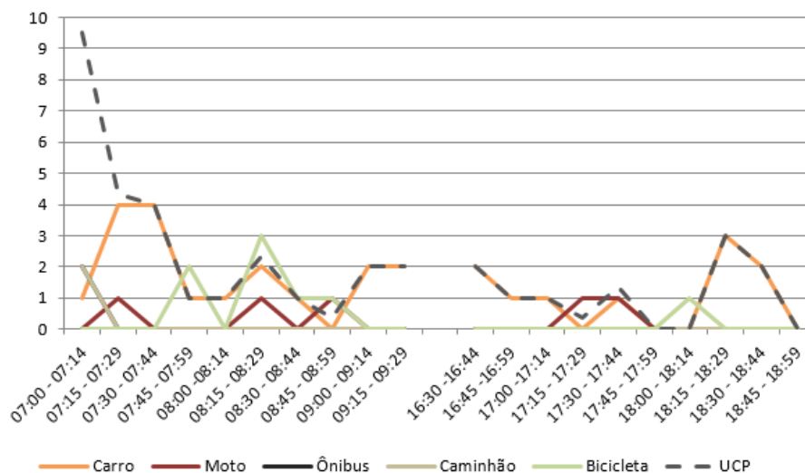
Figura 84 – Gráfico quantidade de veículos para cada intervalo de 15 minutos no M 3
