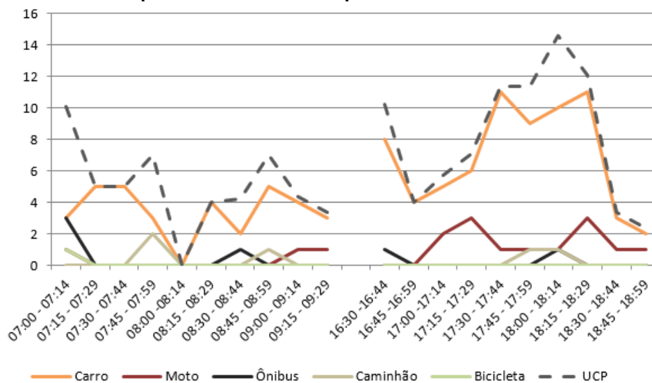
Figura 204 – Gráfico quantidade de veículos para cada intervalo de 15 minutos no M 5
