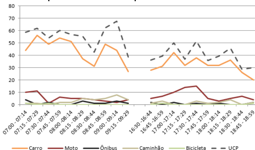
Figura 127 – Gráfico quantidade de veículos para cada intervalo de 15 minutos no M 1
