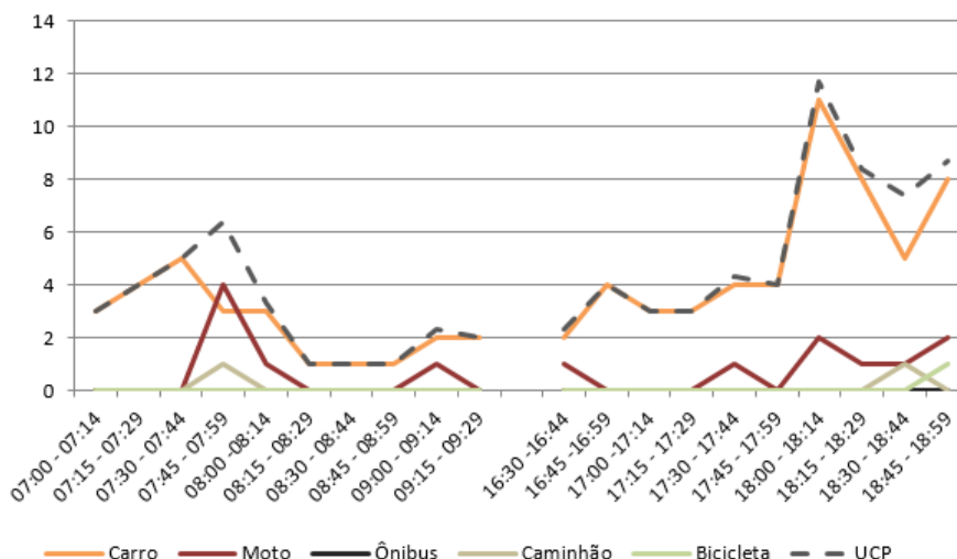
Figura 87 – Gráfico quantidade de veículos para cada intervalo de 15 minutos no M 6
