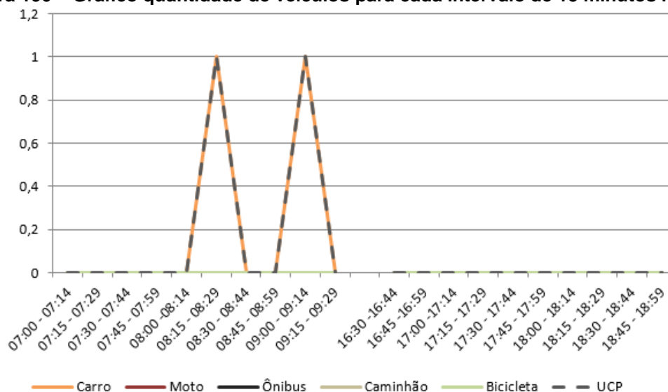
Figura 190 – Gráfico quantidade de veículos para cada intervalo de 15 minutos no M 6
