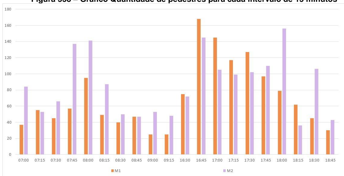
Figura 338 – Gráfico Quantidade de pedestres para cada intervalo de 15 minutos
