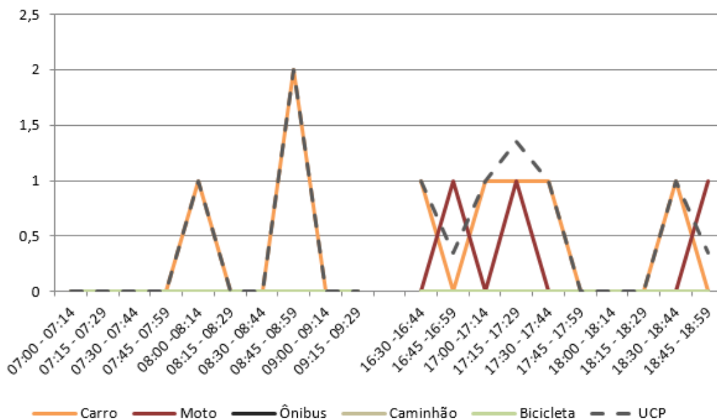
Figura 161 – Gráfico quantidade de veículos para cada intervalo de 15 minutos no M 14
