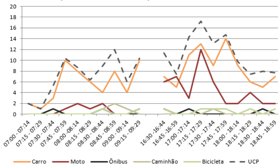
Figura 258 – Gráfico quantidade de veículos para cada intervalo de 15 minutos no M 2
