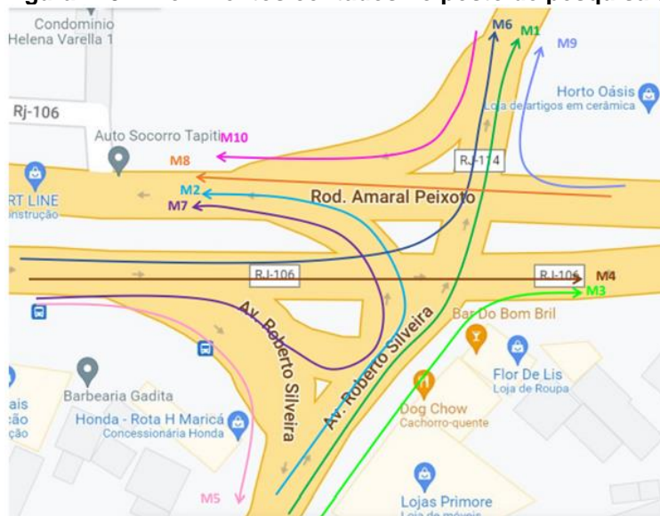
Figura 125 – Movimentos contados no posto de pesquisa 9
