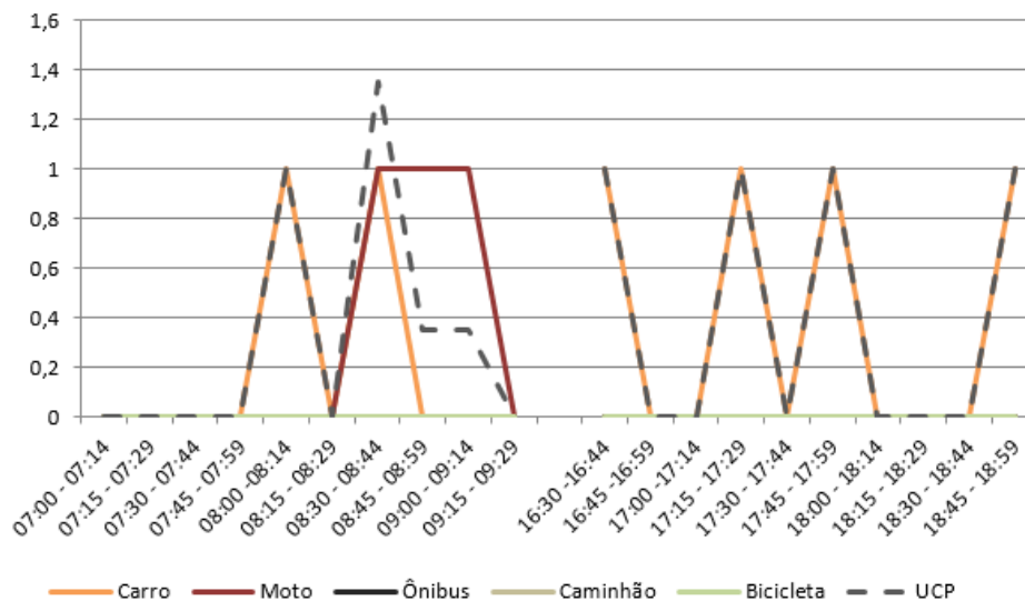
Figura 229 – Gráfico quantidade de veículos para cada intervalo de 15 minutos no M 13
