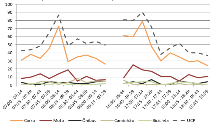
Figura 119 – Gráfico quantidade de veículos para cada intervalo de 15 minutos no M 1
