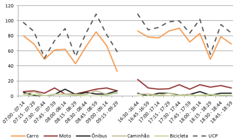
Figura 173 – Gráfico quantidade de veículos para cada intervalo de 15 minutos no M 6
