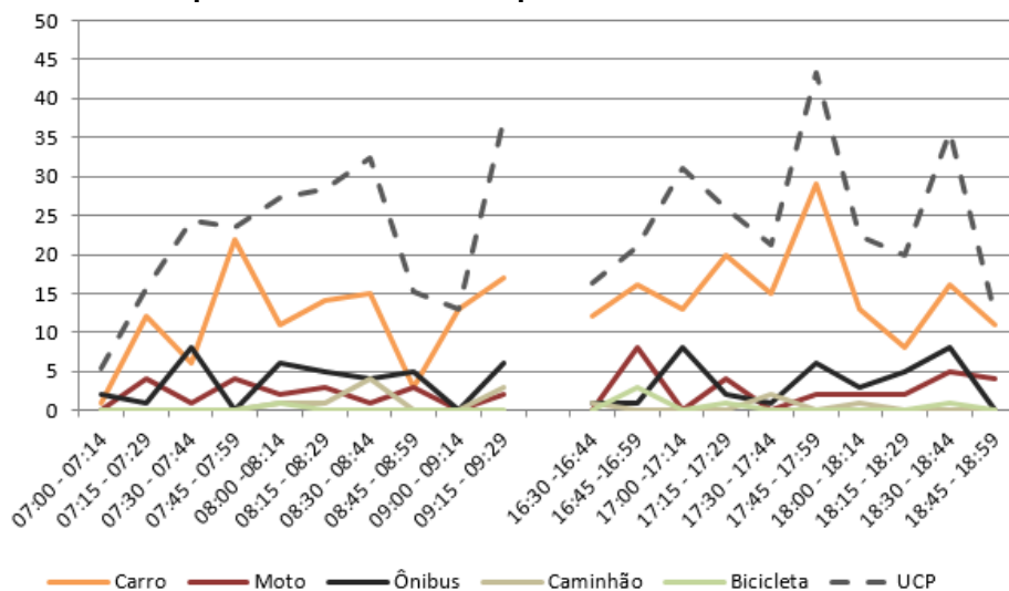
Figura 86 – Gráfico quantidade de veículos para cada intervalo de 15 minutos no M 5
