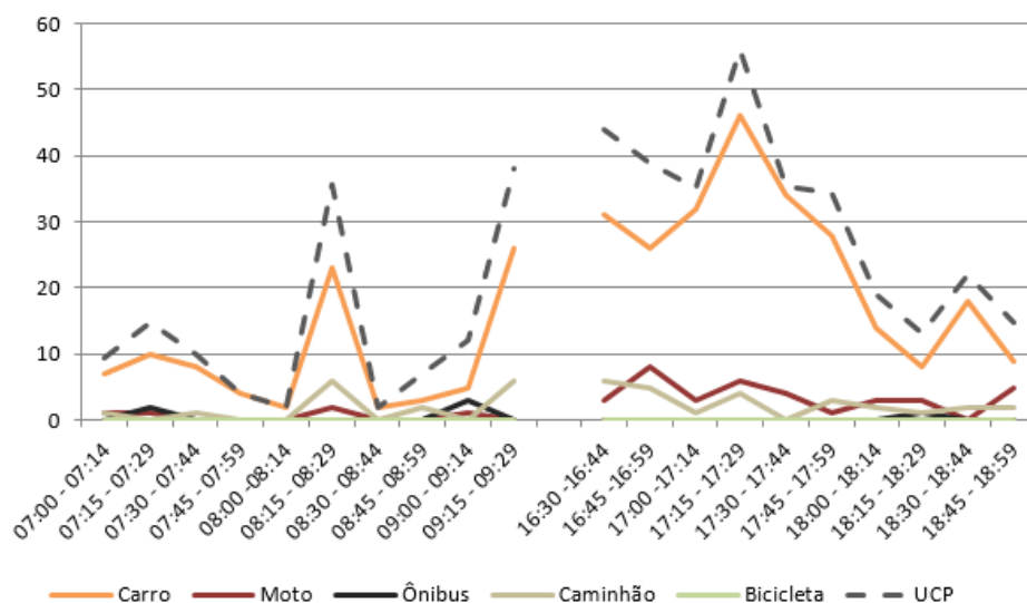
Figura 132 – Gráfico quantidade de veículos para cada intervalo de 15 minutos no M 6
