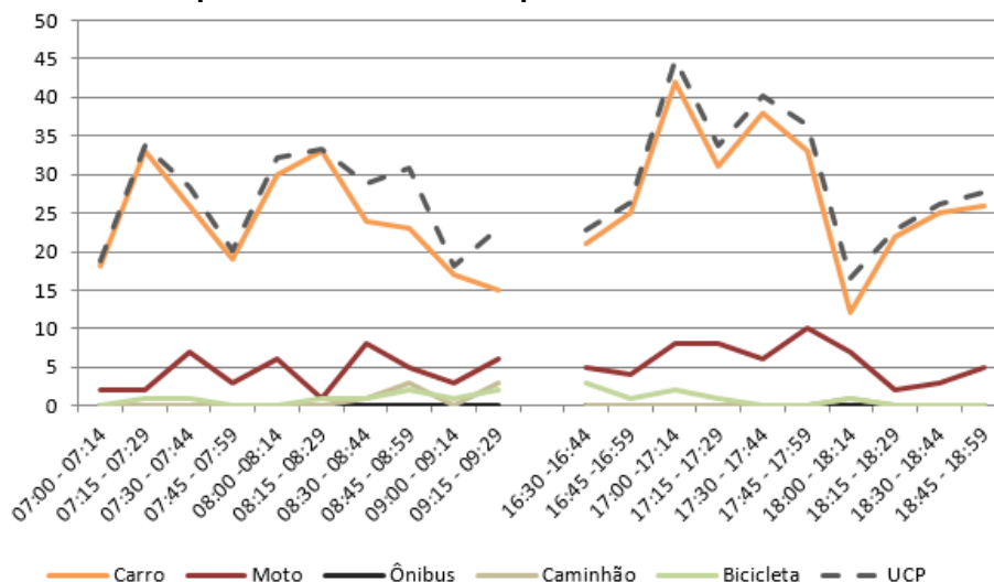
Figura 221 – Gráfico quantidade de veículos para cada intervalo de 15 minutos no M 5
