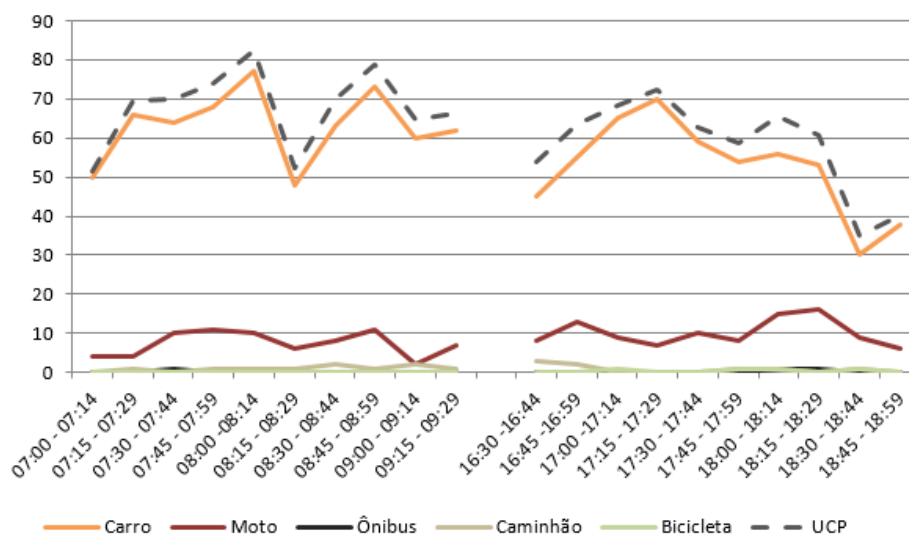
Figura 120 – Gráfico quantidade de veículos para cada intervalo de 15 minutos no M 2
