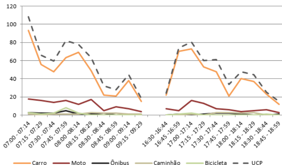
Figura 77 – Gráfico quantidade de veículos para cada intervalo de 15 minutos no M 4
