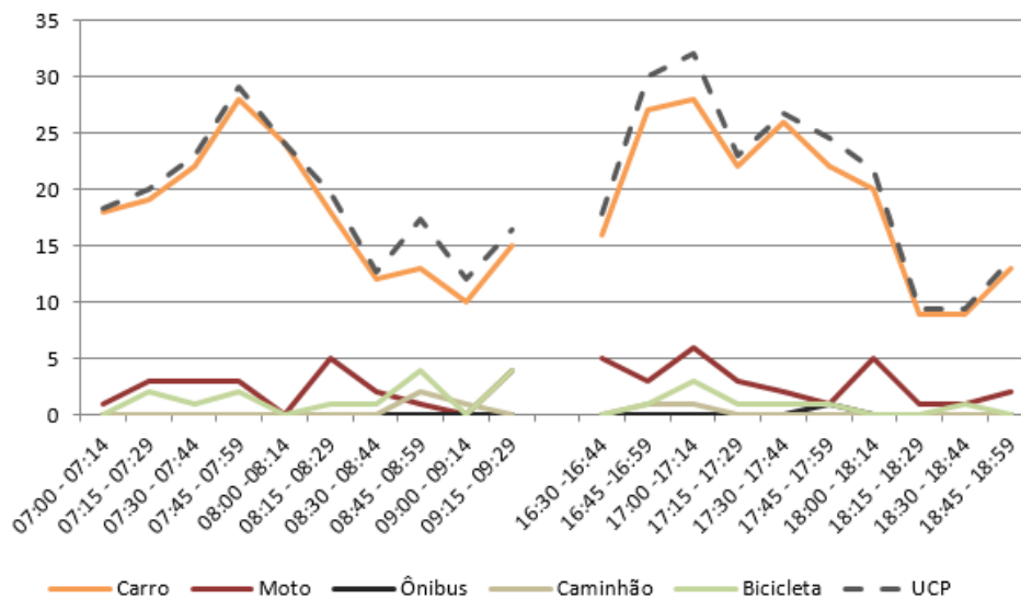
Figura 88 – Gráfico quantidade de veículos para cada intervalo de 15 minutos no M 7
