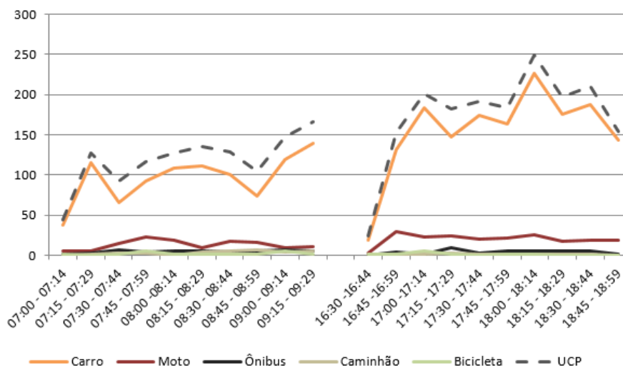
Figura 78 – Gráfico quantidade de veículos para cada intervalo de 15 minutos no M 5
