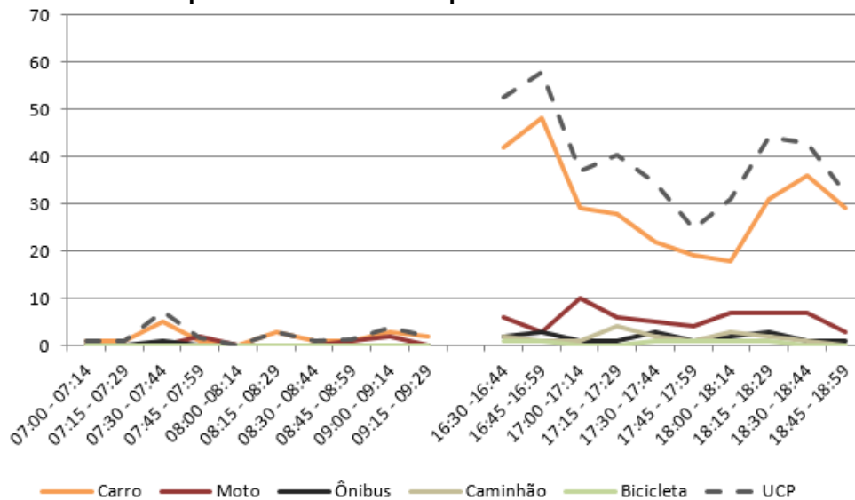
Figura 207 – Gráfico quantidade de veículos para cada intervalo de 15 minutos no M 8
