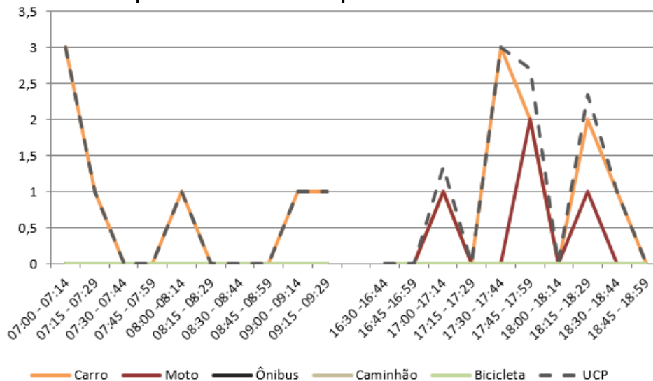
Figura 104 – Gráfico quantidade de veículos para cada intervalo de 15 minutos no M 9
