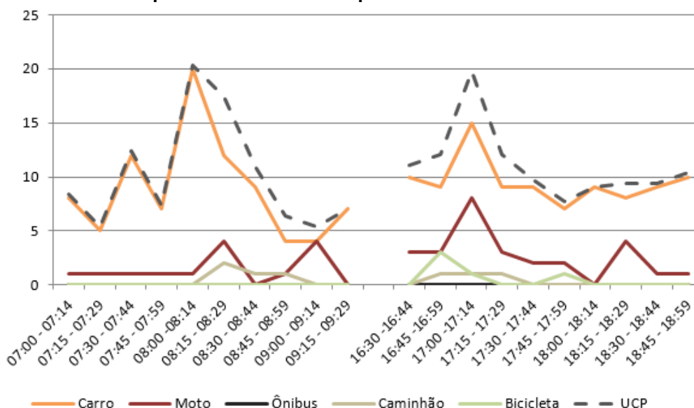
Figura 150 – Gráfico quantidade de veículos para cada intervalo de 15 minutos no M 3
