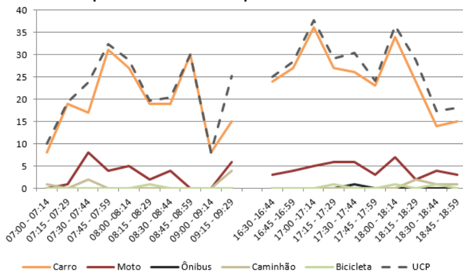
Figura 185 – Gráfico quantidade de veículos para cada intervalo de 15 minutos no M 1
