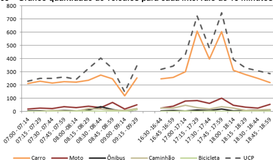
Figura 108 – Gráfico quantidade de veículos para cada intervalo de 15 minutos no M 2
