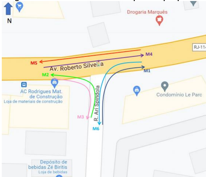
Figura 247 – Movimentos contados no posto de pesquisa 18
