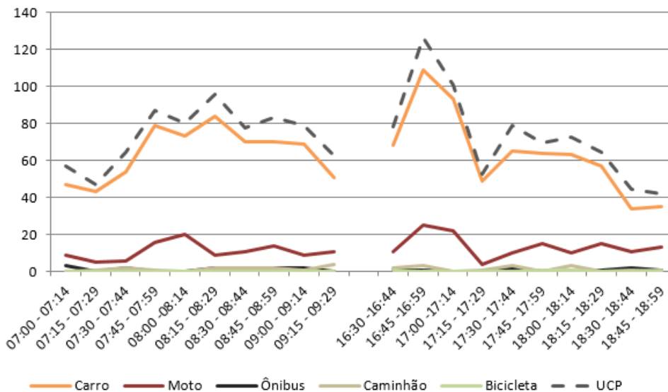
Figura 254 – Gráfico quantidade de veículos para cada intervalo de 15 minutos no M 6
