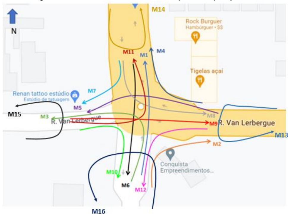
Figura 215 – Movimentos contados no posto de pesquisa 16
