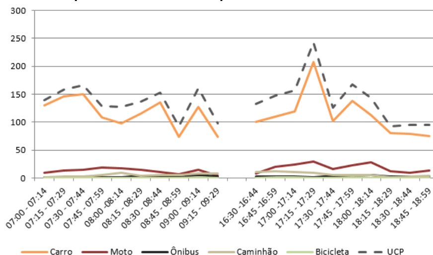
Figura 62 – Gráfico quantidade de veículos para cada intervalo de 15 minutos no M 1
