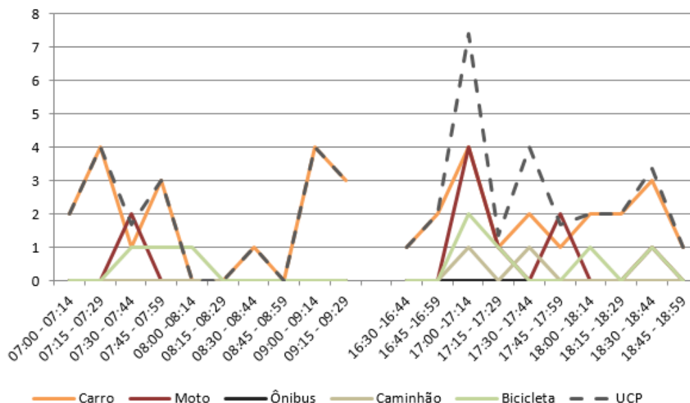
Figura 212 – Gráfico quantidade de veículos para cada intervalo de 15 minutos no M 3
