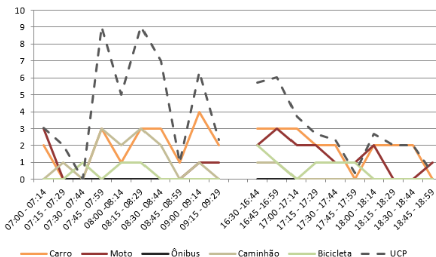
Figura 144 – Gráfico quantidade de veículos para cada intervalo de 15 minutos no M 7
