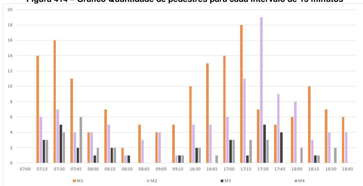
Figura 414 – Gráfico Quantidade de pedestres para cada intervalo de 15 minutos
