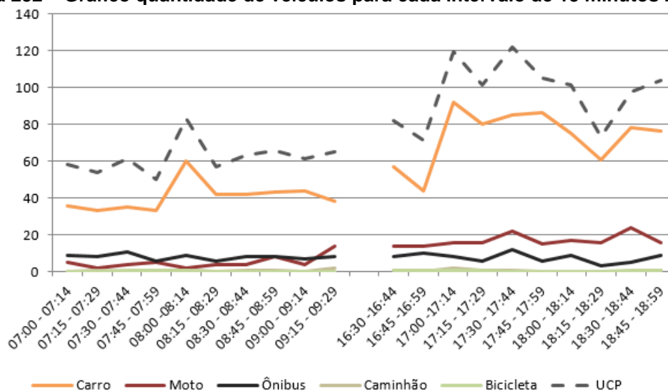
Figura 252 – Gráfico quantidade de veículos para cada intervalo de 15 minutos no M 4
