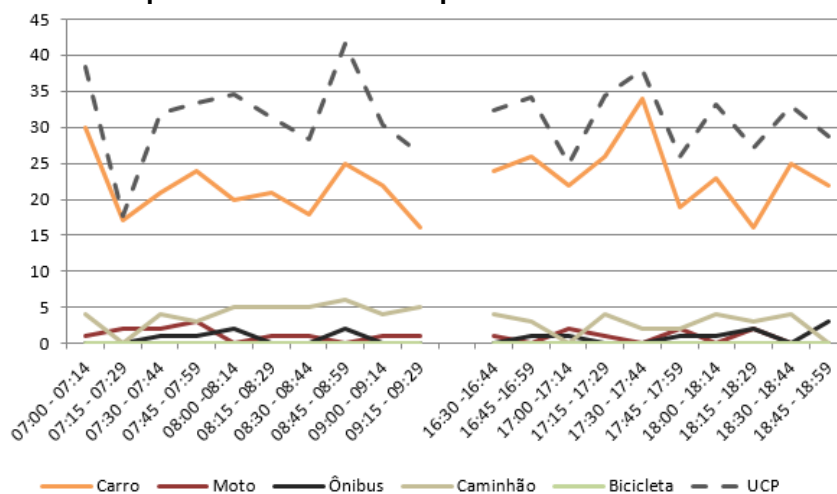
Figura 141 – Gráfico quantidade de veículos para cada intervalo de 15 minutos no M 3
