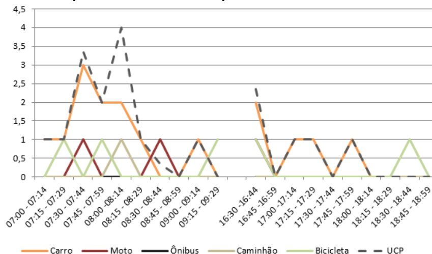
Figura 96 – Gráfico quantidade de veículos para cada intervalo de 15 minutos no M 1
