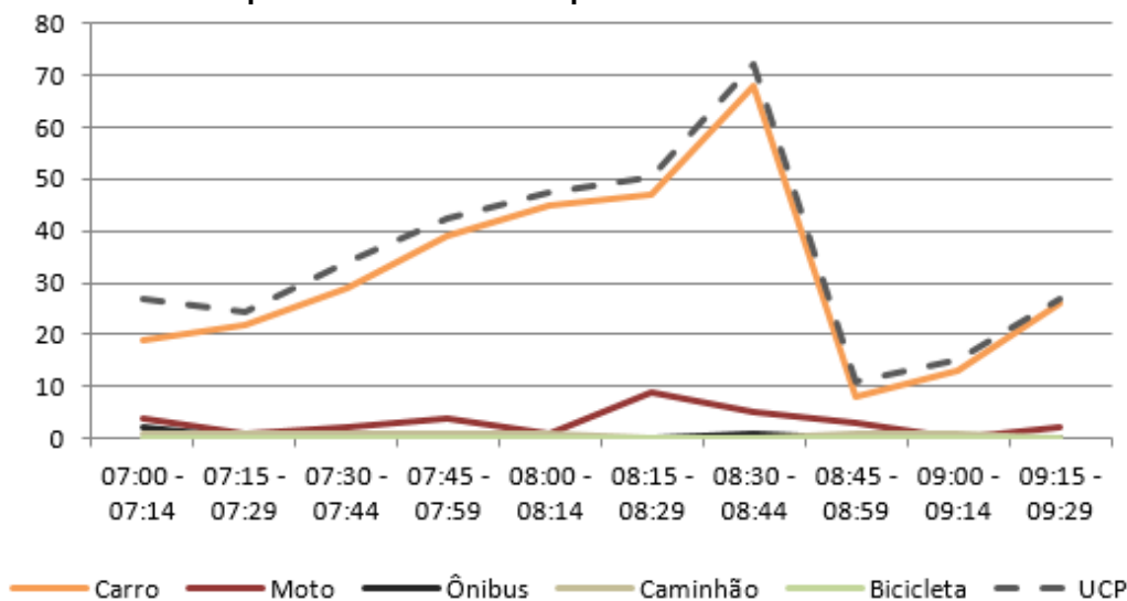
Figura 179 – Gráfico quantidade de veículos para cada intervalo de 15 minutos no M 12
