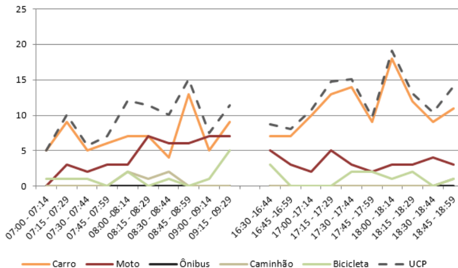
Figura 223 – Gráfico quantidade de veículos para cada intervalo de 15 minutos no M 7
