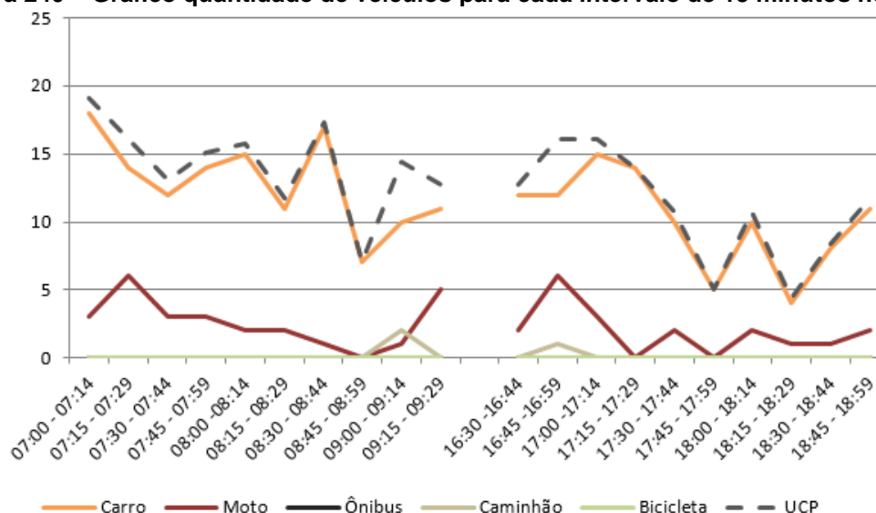
Figura 240 – Gráfico quantidade de veículos para cada intervalo de 15 minutos no M 6
