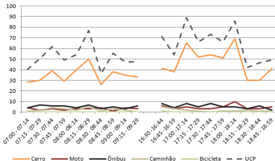
Figura 128 – Gráfico quantidade de veículos para cada intervalo de 15 minutos no M 2
