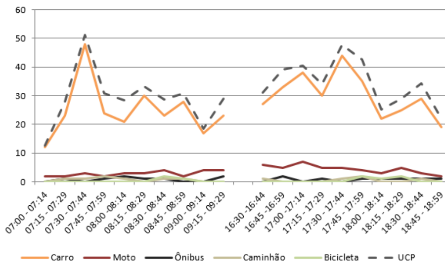
Figura 82 – Gráfico quantidade de veículos para cada intervalo de 15 minutos no M 1
