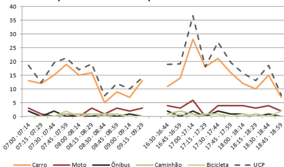
Figura 236 – Gráfico quantidade de veículos para cada intervalo de 15 minutos no M 2
