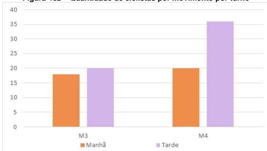
Figura 462 – Quantidade de ciclistas por movimento por turno
