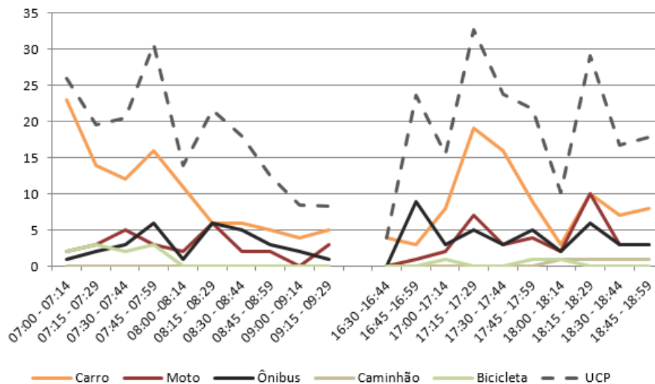
Figura 75 – Gráfico quantidade de veículos para cada intervalo de 15 minutos no M 2
