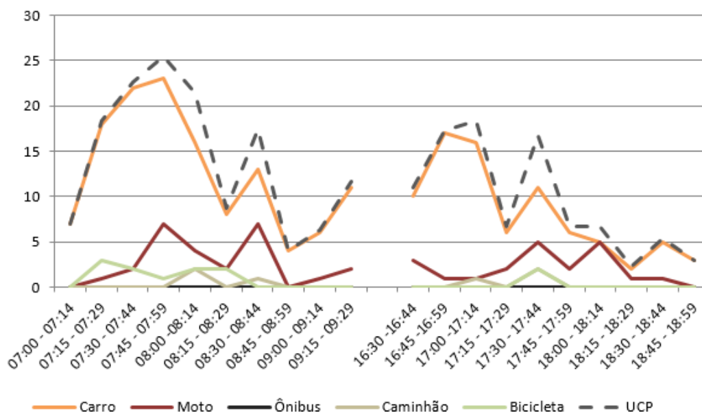
Figura 192 – Gráfico quantidade de veículos para cada intervalo de 15 minutos no M 8
