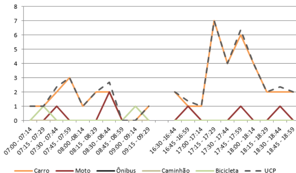
Figura 218 – Gráfico quantidade de veículos para cada intervalo de 15 minutos no M 2
