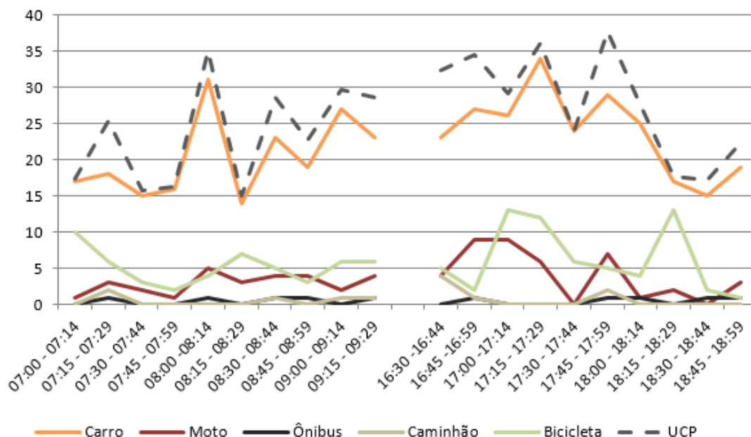
Figura 188 – Gráfico quantidade de veículos para cada intervalo de 15 minutos no M 4
