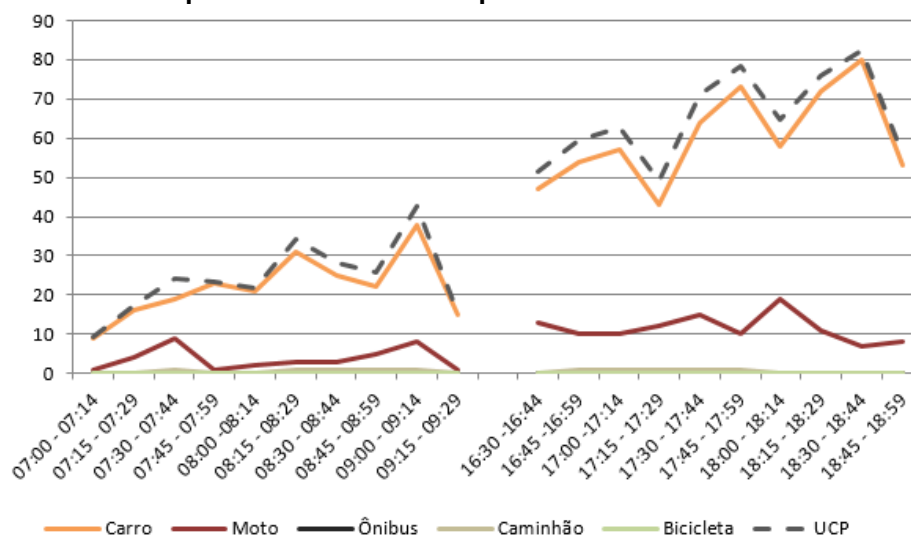
Figura 100 – Gráfico quantidade de veículos para cada intervalo de 15 minutos no M 5
