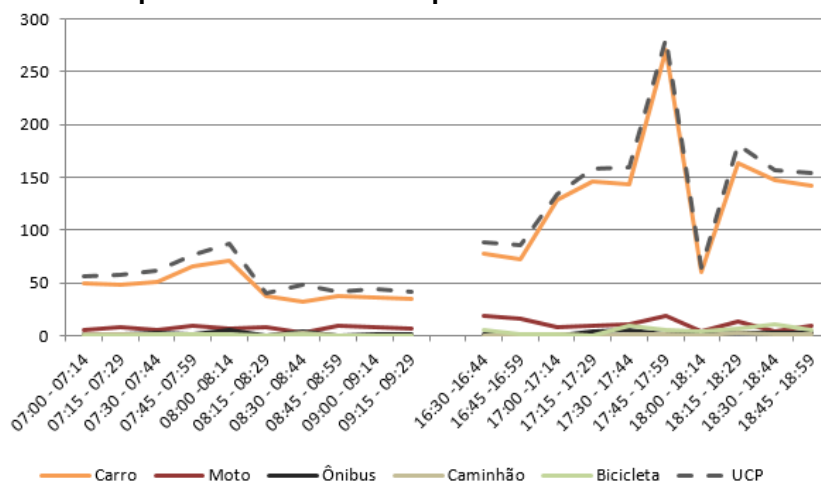
Figura 115 – Gráfico quantidade de veículos para cada intervalo de 15 minutos no M 4
