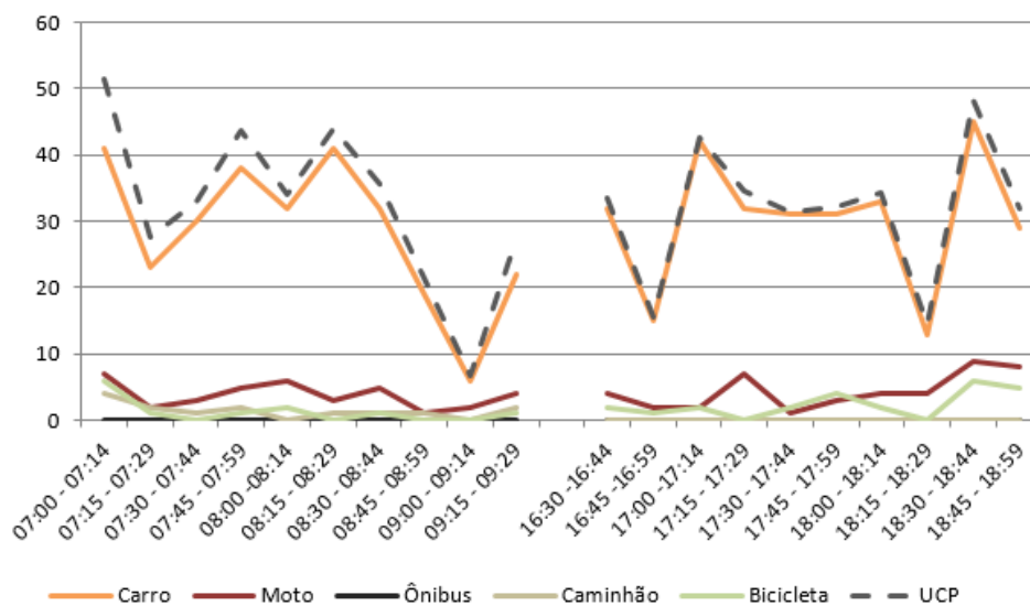
Figura 191 – Gráfico quantidade de veículos para cada intervalo de 15 minutos no M 7
