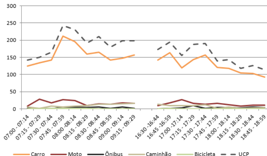
Figura 134 – Gráfico quantidade de veículos para cada intervalo de 15 minutos no M 8
