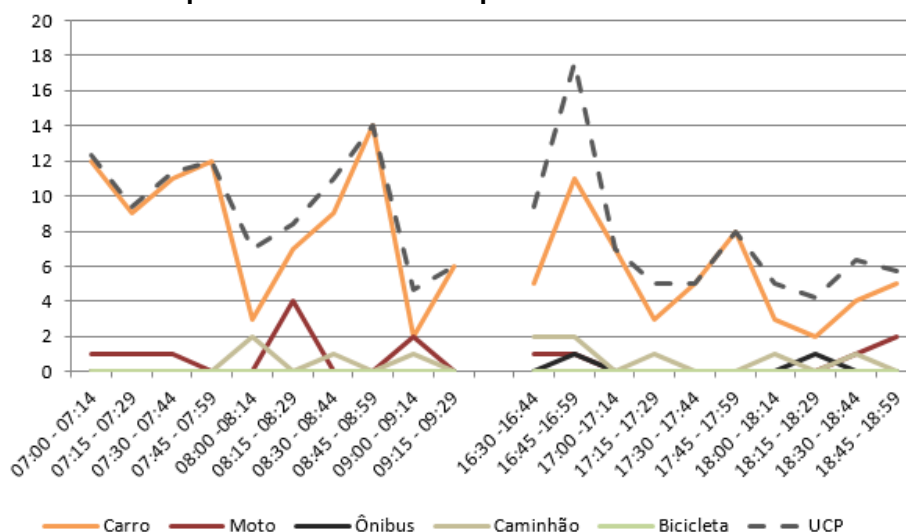
Figura 243 – Gráfico quantidade de veículos para cada intervalo de 15 minutos no M 9
