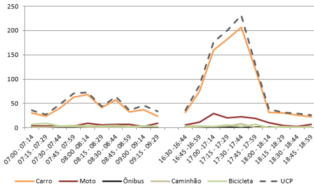
Figura 267 – Gráfico quantidade de veículos para cada intervalo de 15 minutos no M 3
