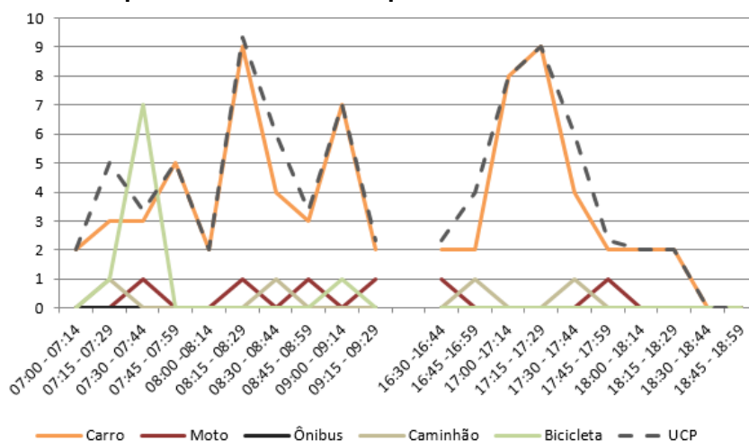
Figura 63 – Gráfico quantidade de veículos para cada intervalo de 15 minutos no M 2
