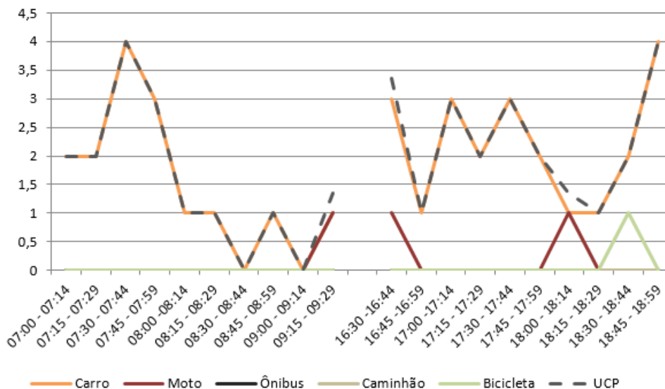
Figura 90 – Gráfico quantidade de veículos para cada intervalo de 15 minutos no M 9
