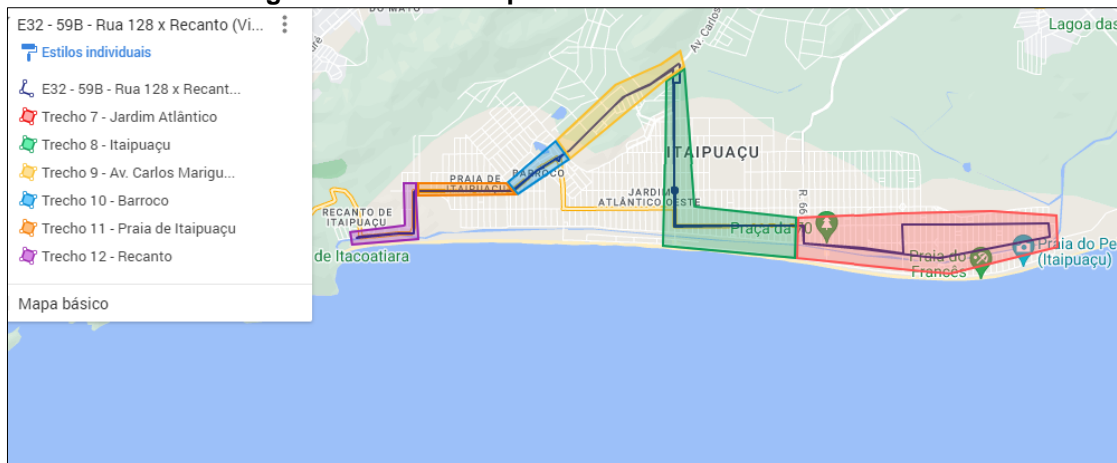
Figura 612 – Divisão por trechos – Linha E32 Volta
