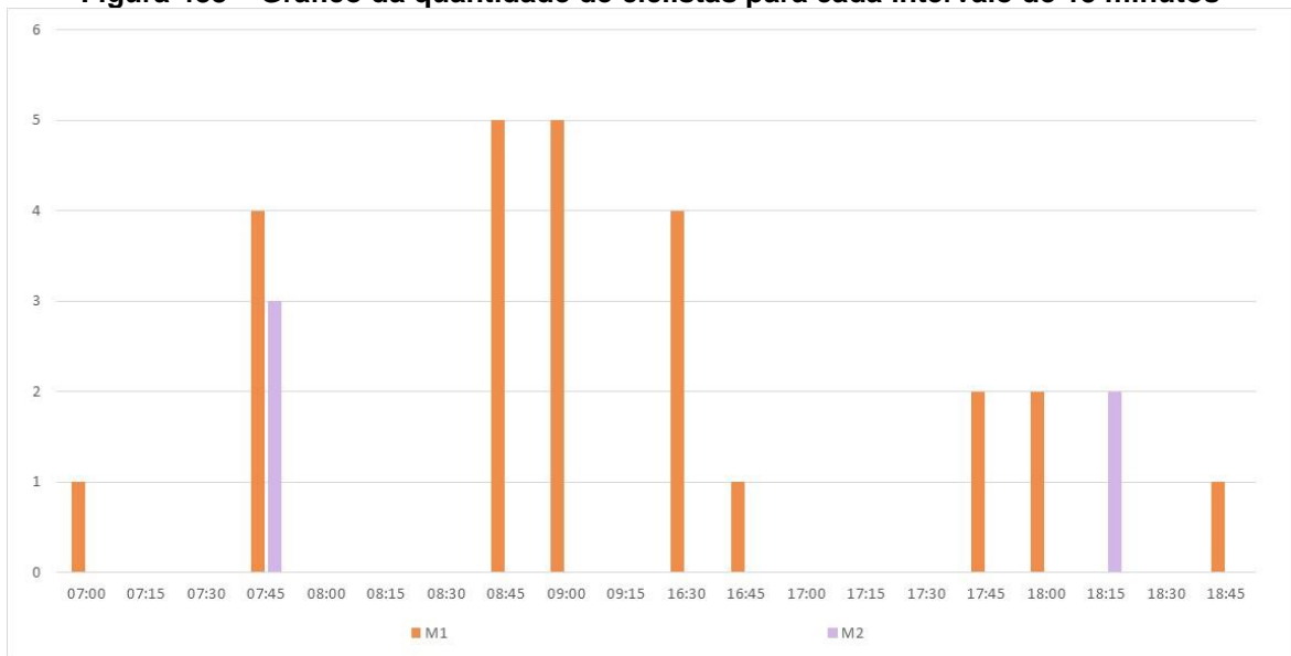
Figura 488 – Gráfico da quantidade de ciclistas para cada intervalo de 15 minutos
