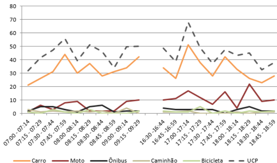
Figura 121 – Gráfico quantidade de veículos para cada intervalo de 15 minutos no M 3
