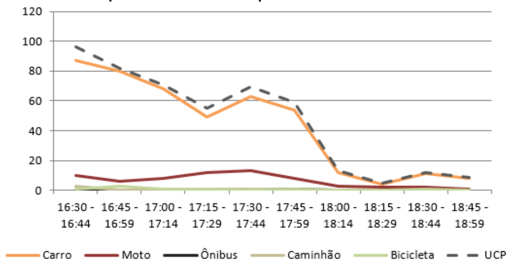
Figura 182 – Gráfico quantidade de veículos para cada intervalo de 15 minutos no M 15
