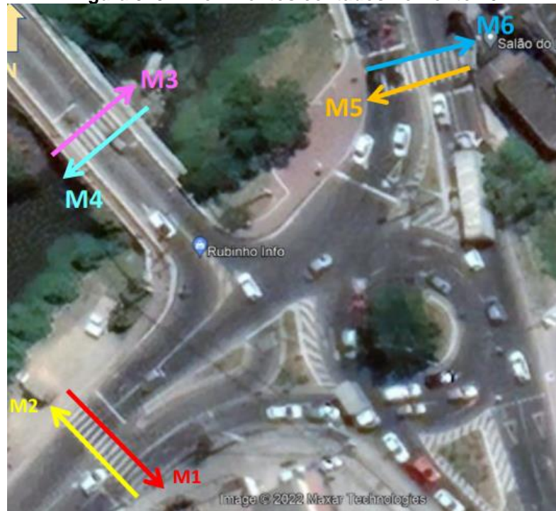
Figura 379 – Movimentos contados no Ponto 20
