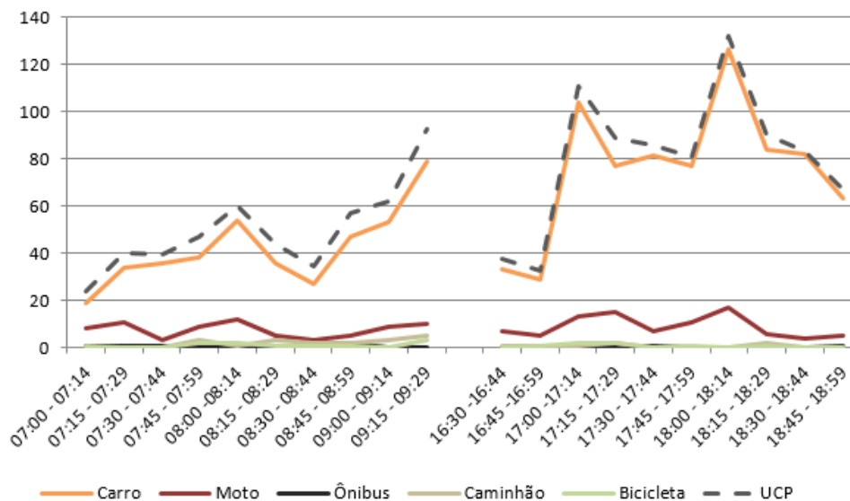
Figura 76 – Gráfico quantidade de veículos para cada intervalo de 15 minutos no M 3
