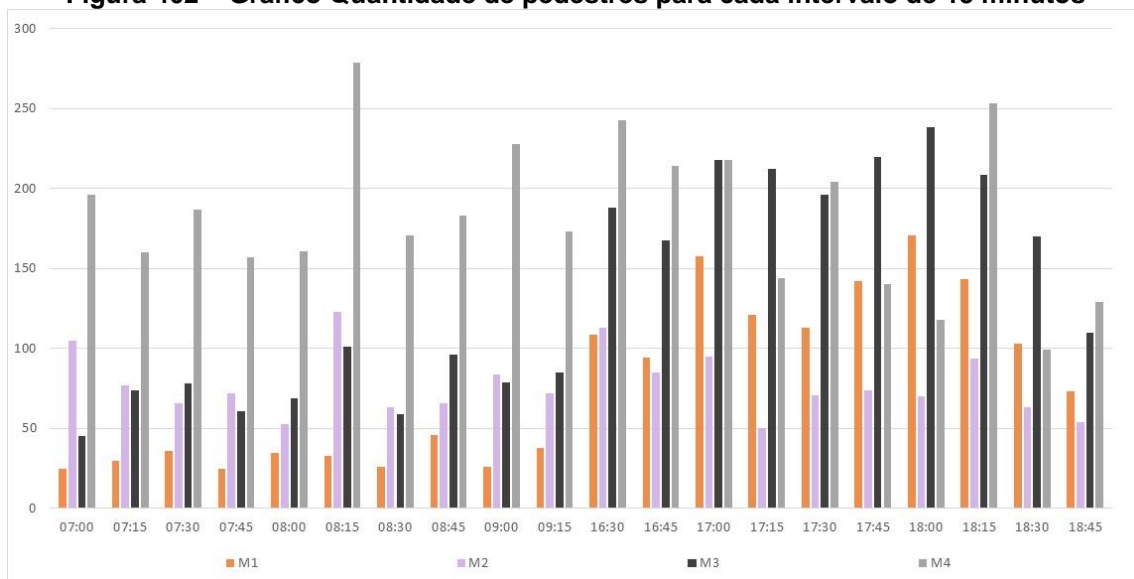
Figura 402 – Gráfico Quantidade de pedestres para cada intervalo de 15 minutos
