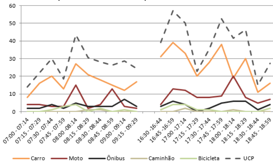
Figura 251 – Gráfico quantidade de veículos para cada intervalo de 15 minutos no M 3
