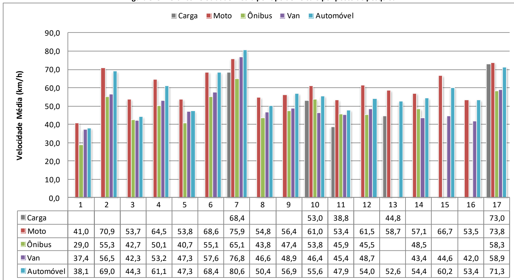
Figura 529 – Gráfico velocidade média por tipo de veículo por posto de pesquisa
