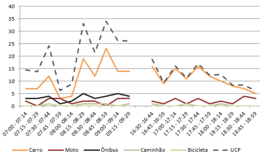
Figura 219 – Gráfico quantidade de veículos para cada intervalo de 15 minutos no M 3
