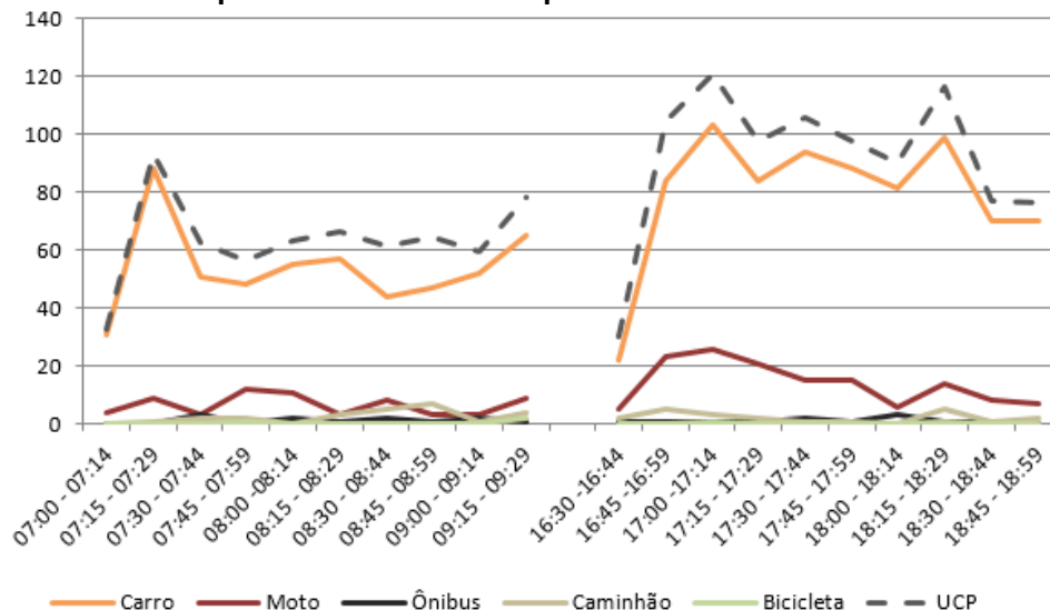
Figura 79 – Gráfico quantidade de veículos para cada intervalo de 15 minutos no M 6
