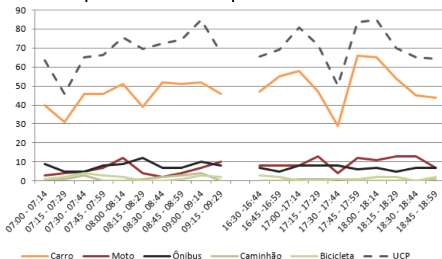
Figura 253 – Gráfico quantidade de veículos para cada intervalo de 15 minutos no M 5
