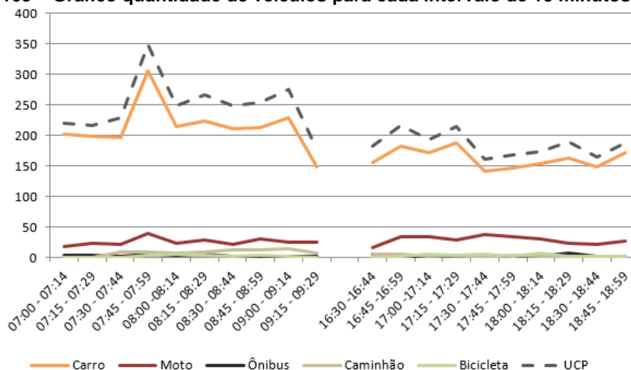
Figura 109 – Gráfico quantidade de veículos para cada intervalo de 15 minutos no M 3
