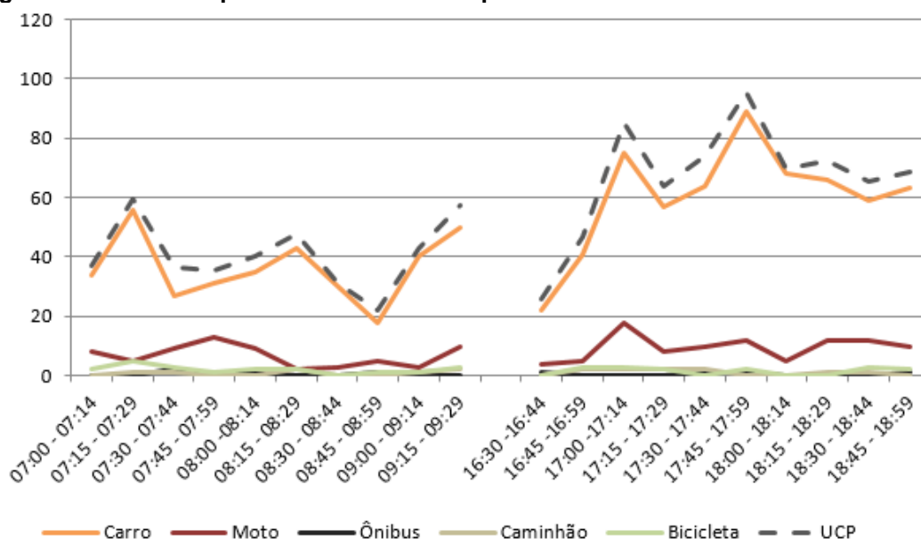
Figura 210 – Gráfico quantidade de veículos para cada intervalo de 15 minutos no M 1
