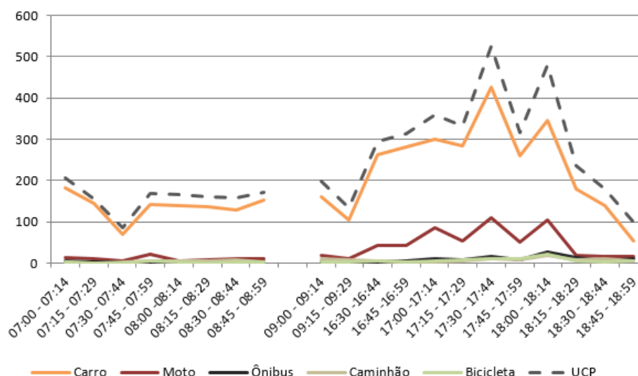
Figura 168 – Gráfico quantidade de veículos para cada intervalo de 15 minutos no M 1
