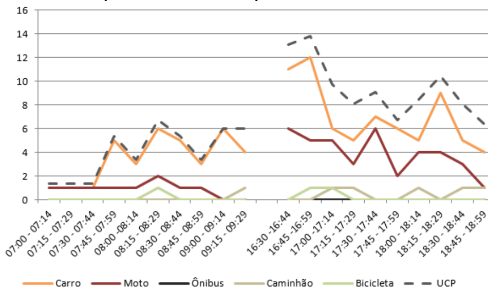
Figura 149 – Gráfico quantidade de veículos para cada intervalo de 15 minutos no M 2
