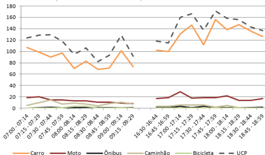
Figura 71 – Gráfico quantidade de veículos para cada intervalo de 15 minutos no M 3
