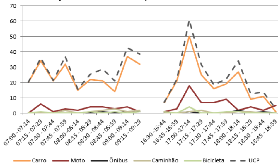
Figura 211 – Gráfico quantidade de veículos para cada intervalo de 15 minutos no M 2
