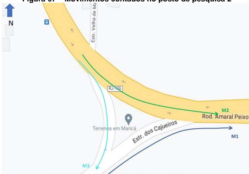
Figura 67 – Movimentos contados no posto de pesquisa 2
