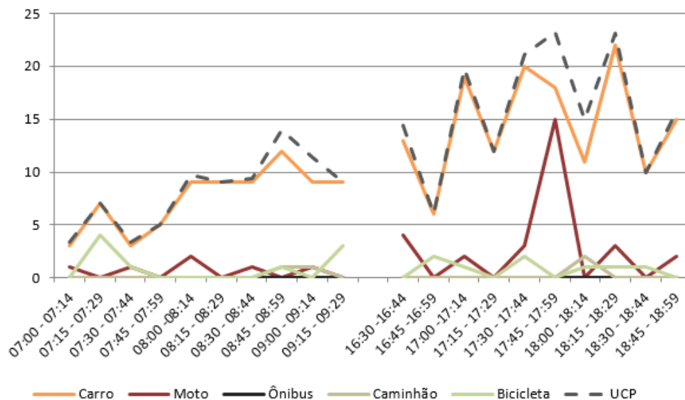
Figura 226 – Gráfico quantidade de veículos para cada intervalo de 15 minutos no M 10
