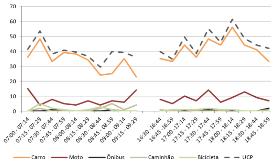
Figura 244 – Gráfico quantidade de veículos para cada intervalo de 15 minutos no M 10
