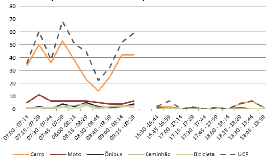
Figura 200 – Gráfico quantidade de veículos para cada intervalo de 15 minutos no M 1
