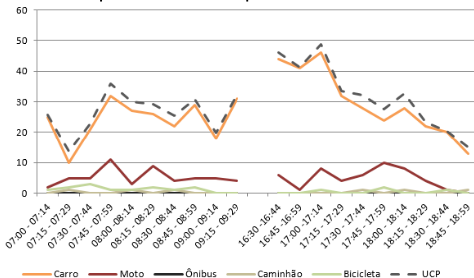
Figura 189 – Gráfico quantidade de veículos para cada intervalo de 15 minutos no M 5
