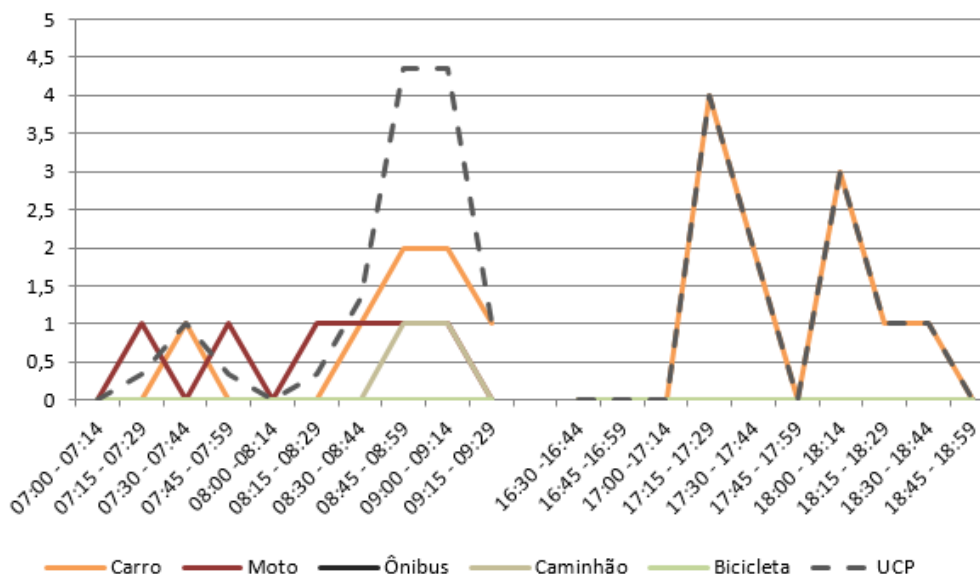
Figura 230 – Gráfico quantidade de veículos para cada intervalo de 15 minutos no M 14
