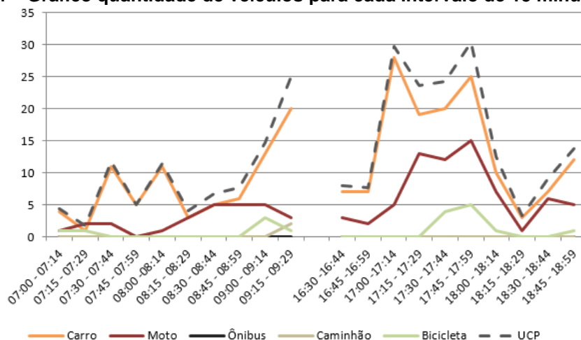
Figura 114 – Gráfico quantidade de veículos para cada intervalo de 15 minutos no M 3
