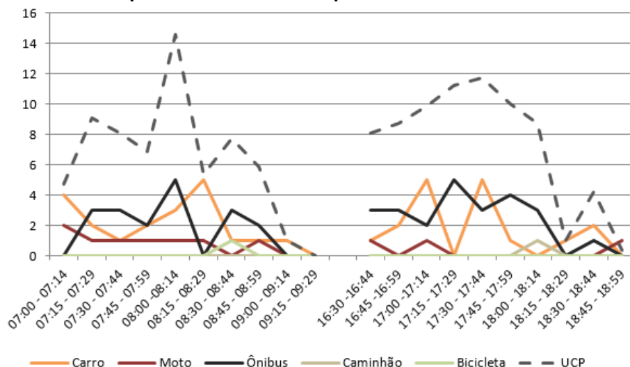
Figura 103 – Gráfico quantidade de veículos para cada intervalo de 15 minutos no M 8
