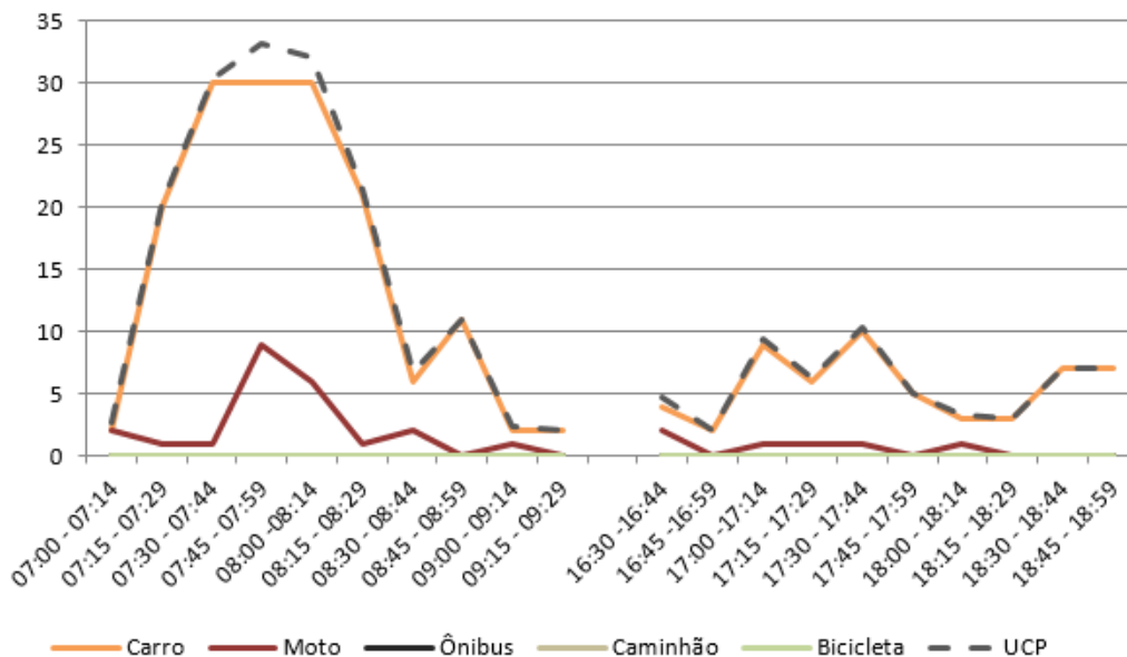
Figura 194 – Gráfico quantidade de veículos para cada intervalo de 15 minutos no M 10
