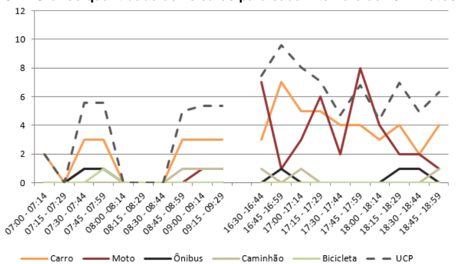
Figura 257 – Gráfico quantidade de veículos para cada intervalo de 15 minutos no M 1
