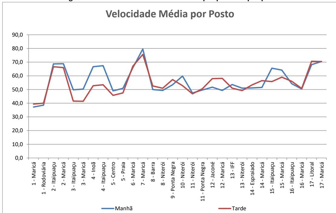
Figura 527 – Gráfico de velocidade média por posto de pesquisa
