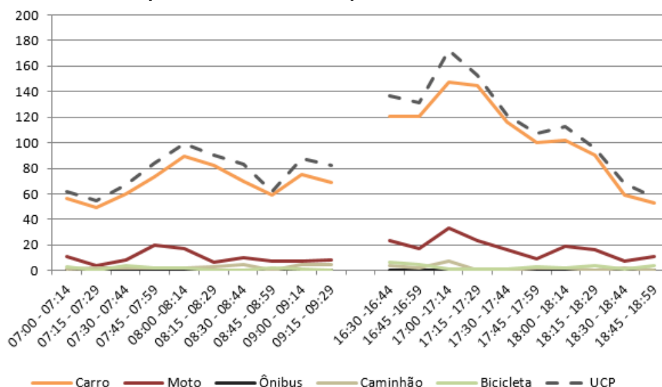
Figura 265 – Gráfico quantidade de veículos para cada intervalo de 15 minutos no M 1
