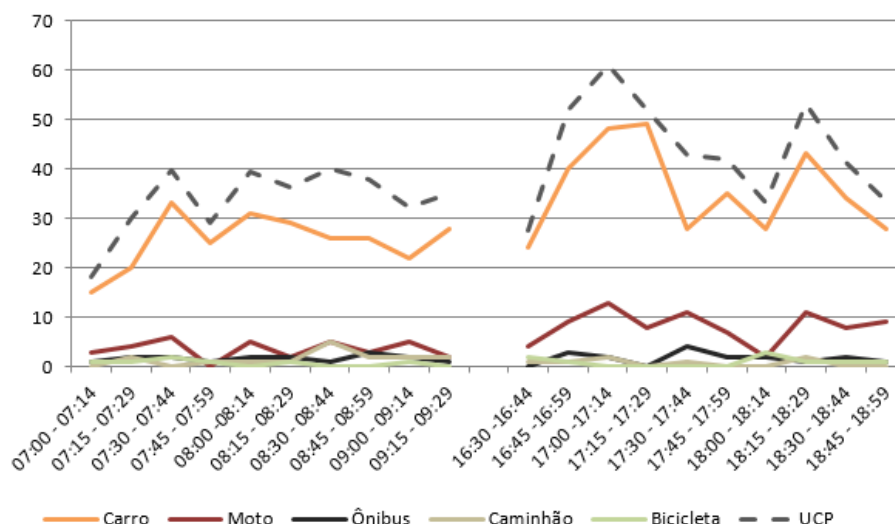
Figura 129 – Gráfico quantidade de veículos para cada intervalo de 15 minutos no M 3
