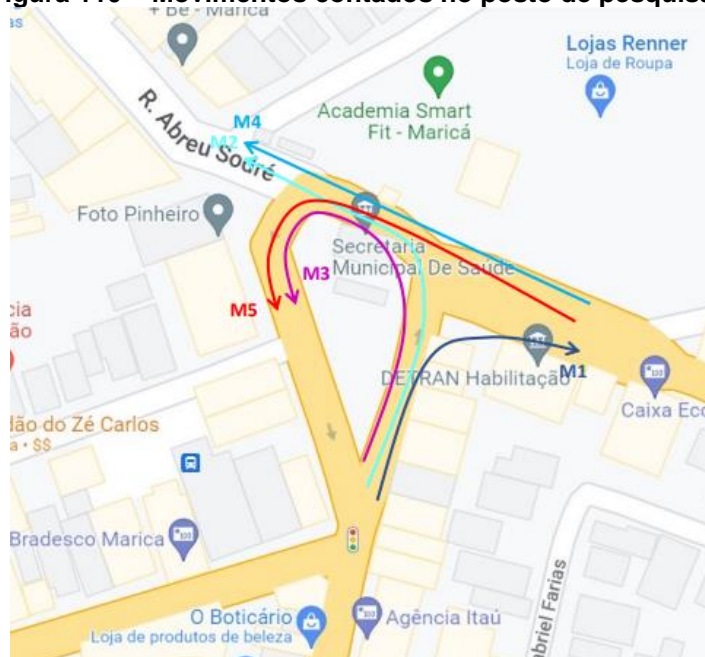
Figura 110 – Movimentos contados no posto de pesquisa 7
