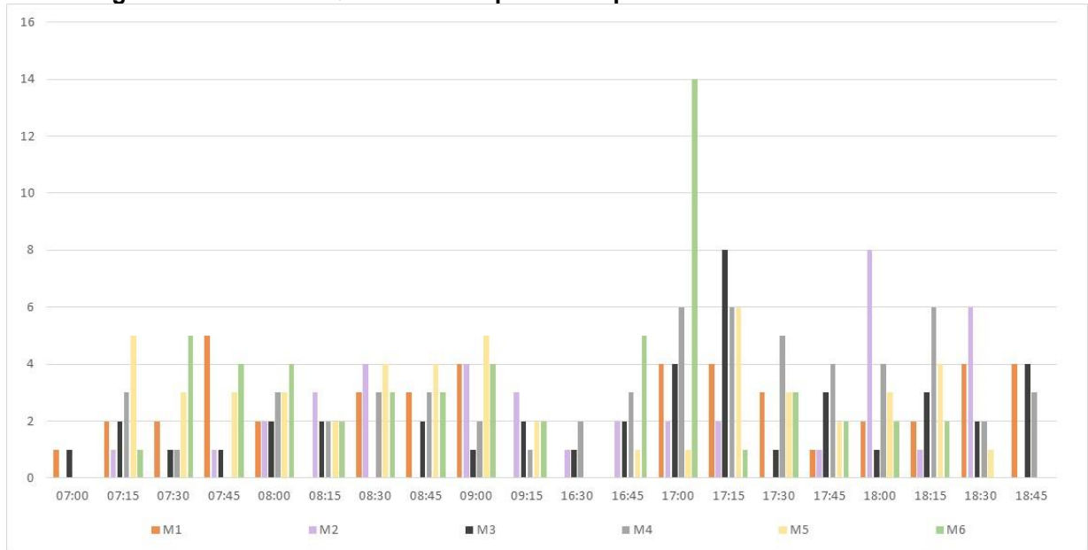
Figura 342 – Gráfico Quantidade de pedestres para cada intervalo de 15 minutos
