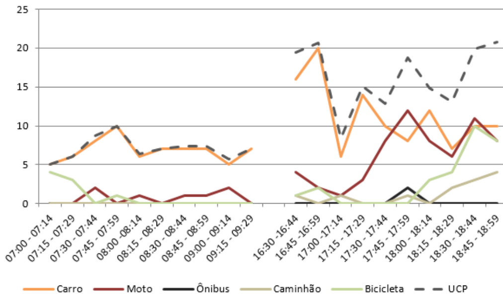
Figura 268 – Gráfico quantidade de veículos para cada intervalo de 15 minutos no M 4
