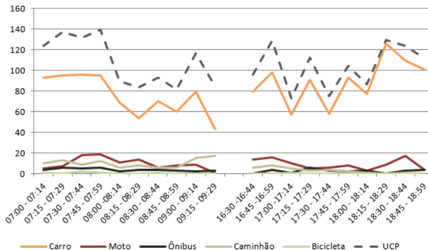
Figura 64 – Gráfico quantidade de veículos para cada intervalo de 15 minutos no M 3
