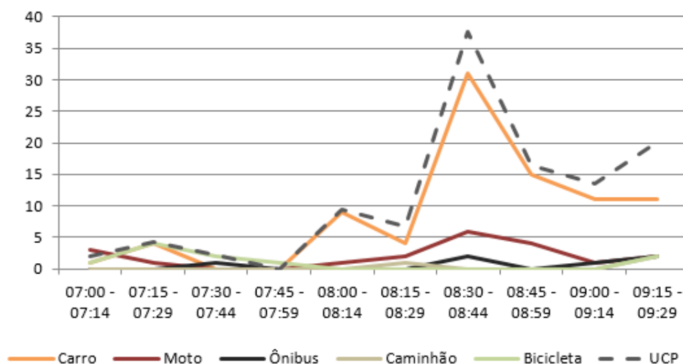
Figura 171 – Gráfico quantidade de veículos para cada intervalo de 15 minutos no M 4
