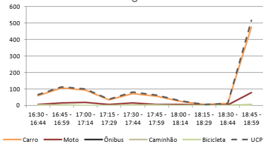
Figura 181 – Gráfico quantidade de veículos para cada intervalo de 15 minutos no M 14
