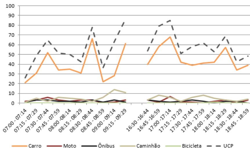
Figura 142 – Gráfico quantidade de veículos para cada intervalo de 15 minutos no M 5
