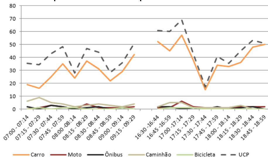
Figura 140 – Gráfico quantidade de veículos para cada intervalo de 15 minutos no M 2
