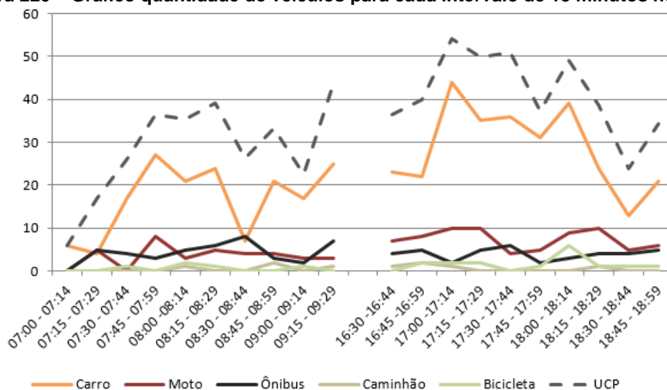
Figura 220 – Gráfico quantidade de veículos para cada intervalo de 15 minutos no M 4
