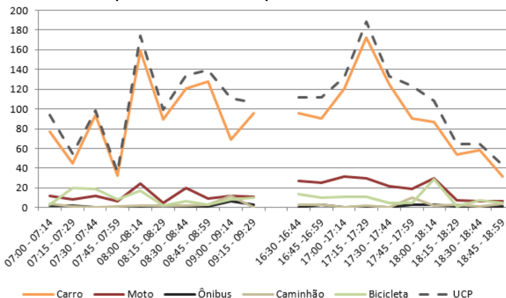
Figura 176 – Gráfico quantidade de veículos para cada intervalo de 15 minutos no M 9
