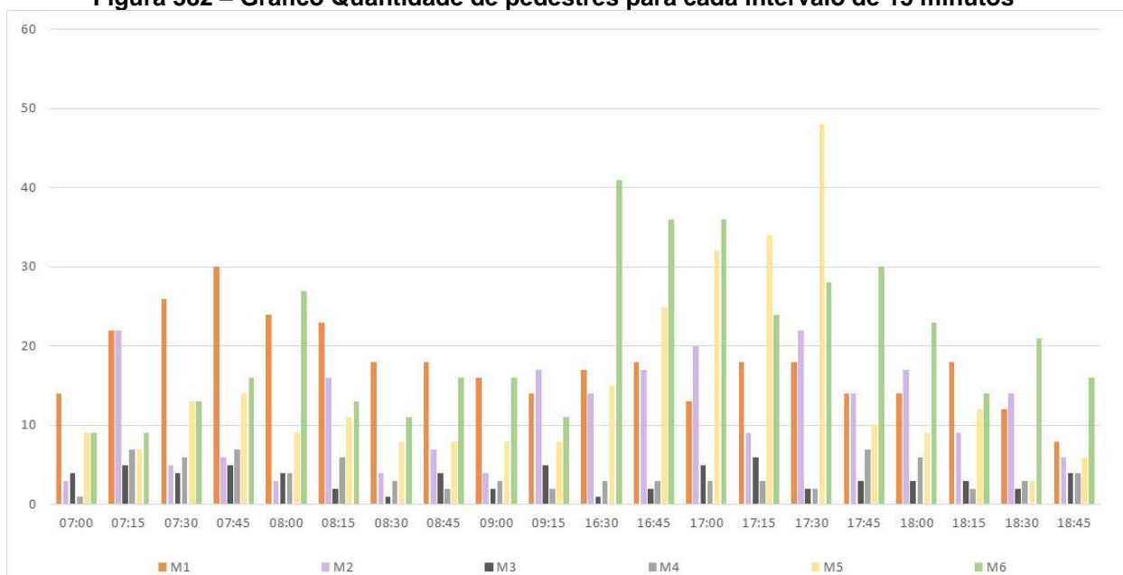
Figura 382 – Gráfico Quantidade de pedestres para cada intervalo de 15 minutos
