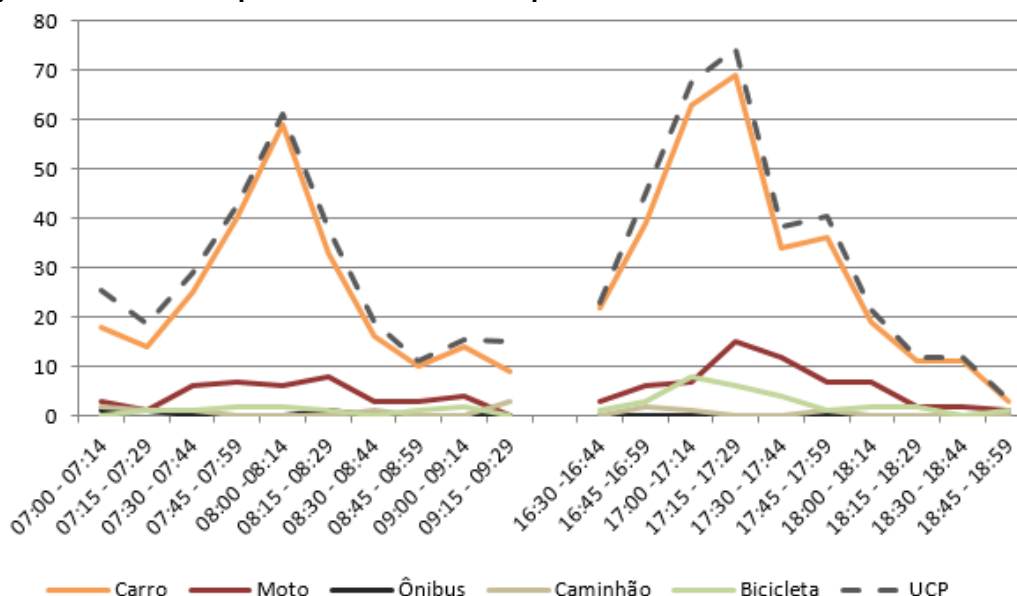
Figura 195 – Gráfico quantidade de veículos para cada intervalo de 15 minutos no M 11
