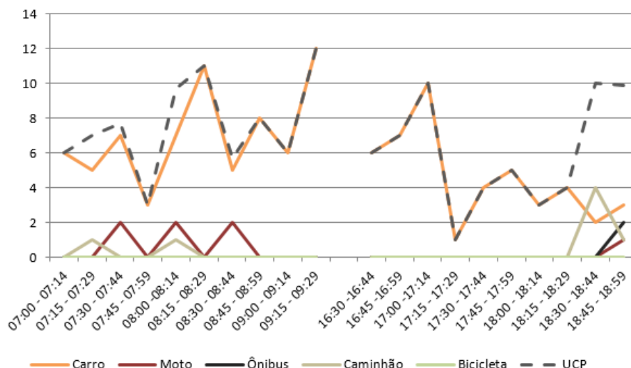
Figura 122 – Gráfico quantidade de veículos para cada intervalo de 15 minutos no M 4
