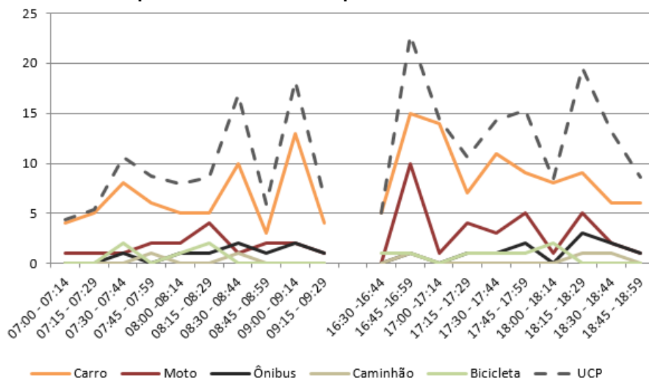
Figura 156 – Gráfico quantidade de veículos para cada intervalo de 15 minutos no M 9
