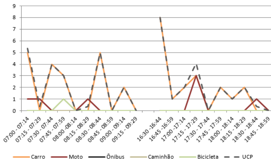
Figura 97 – Gráfico quantidade de veículos para cada intervalo de 15 minutos no M 2
