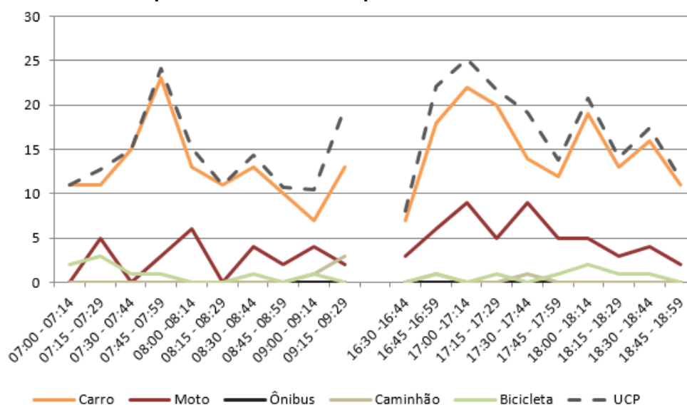
Figura 239 – Gráfico quantidade de veículos para cada intervalo de 15 minutos no M 5
