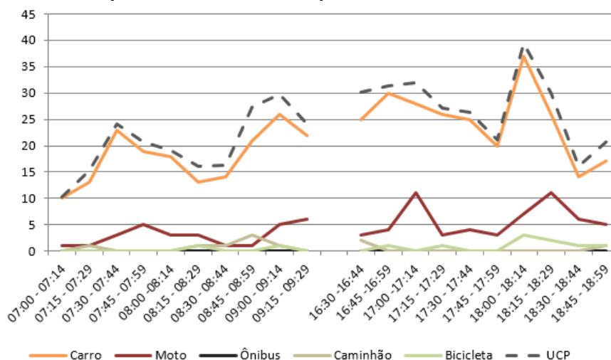
Figura 217 – Gráfico quantidade de veículos para cada intervalo de 15 minutos no M 1
