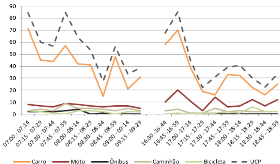
Figura 177 – Gráfico quantidade de veículos para cada intervalo de 15 minutos no M 10
