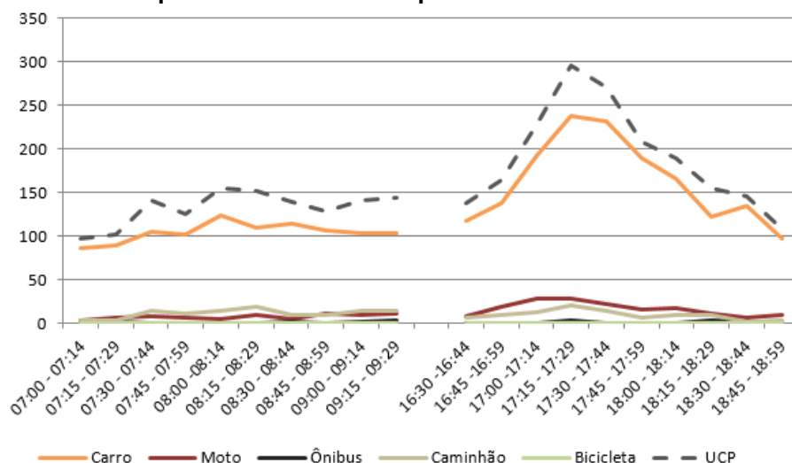
Figura 130 – Gráfico quantidade de veículos para cada intervalo de 15 minutos no M 4
