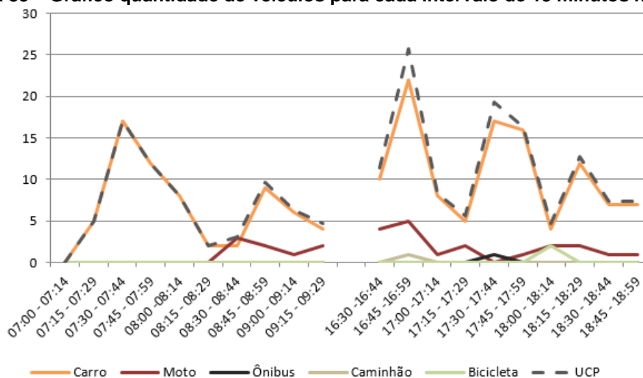
Figura 85 – Gráfico quantidade de veículos para cada intervalo de 15 minutos no M 4
