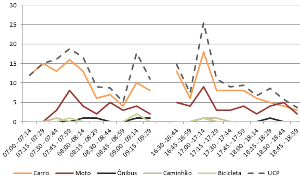
Figura 262 – Gráfico quantidade de veículos para cada intervalo de 15 minutos no M 6
