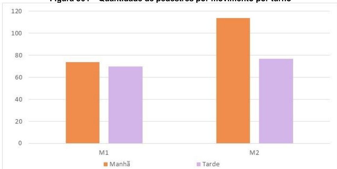
Figura 364 – Quantidade de pedestres por movimento por turno
