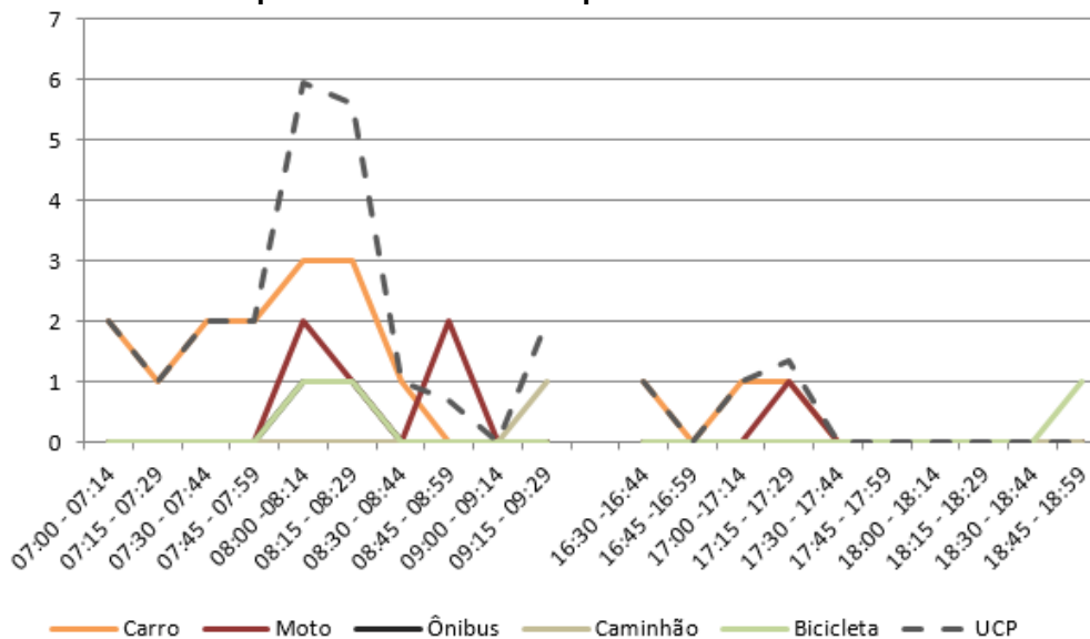
Figura 261 – Gráfico quantidade de veículos para cada intervalo de 15 minutos no M 5
