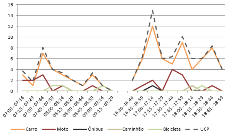
Figura 83 – Gráfico quantidade de veículos para cada intervalo de 15 minutos no M 2
