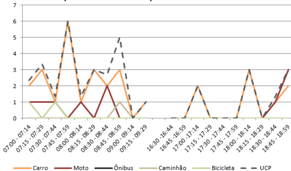
Figura 66 – Gráfico quantidade de veículos para cada intervalo de 15 minutos no M 5
