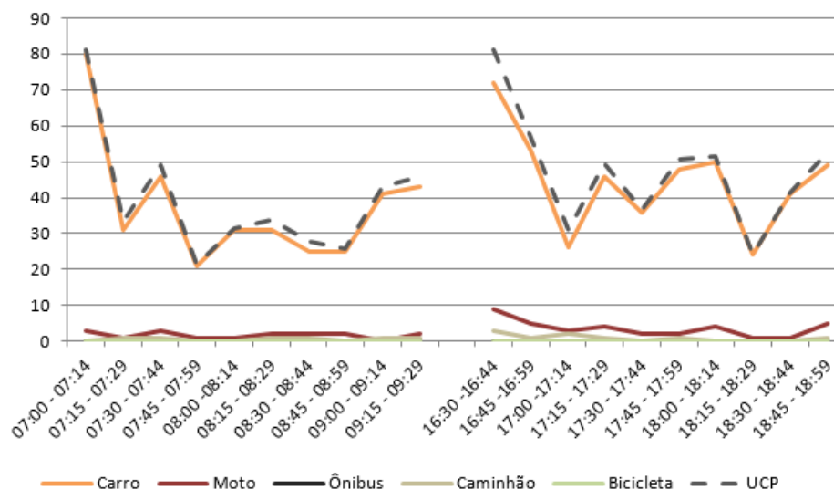
Figura 174 – Gráfico quantidade de veículos para cada intervalo de 15 minutos no M 7
