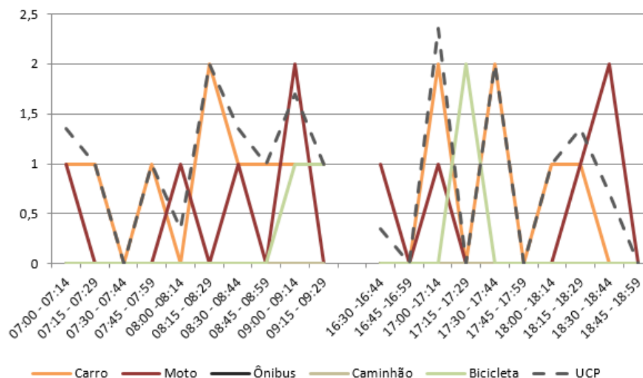
Figura 260 – Gráfico quantidade de veículos para cada intervalo de 15 minutos no M 4
