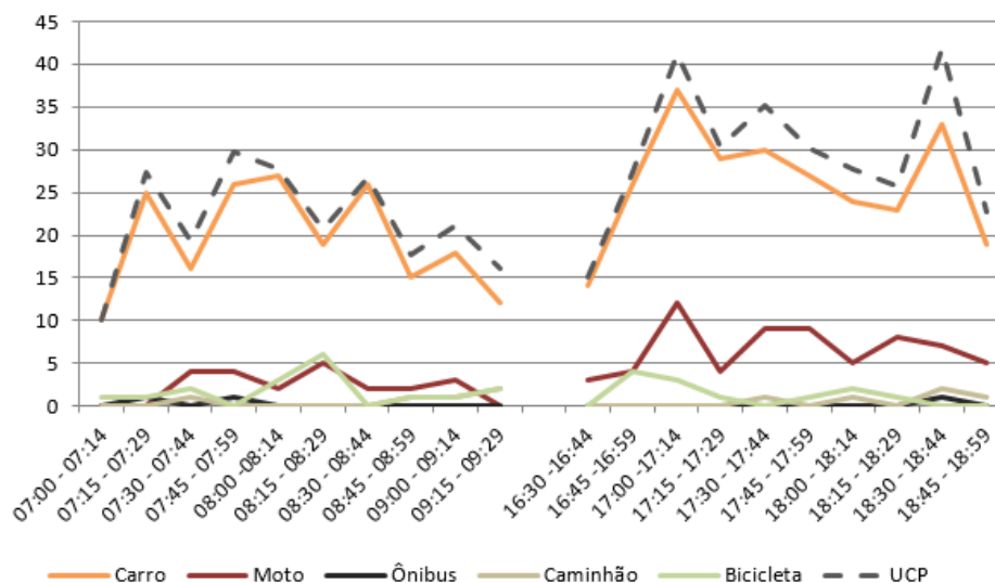
Figura 225 – Gráfico quantidade de veículos para cada intervalo de 15 minutos no M 9
