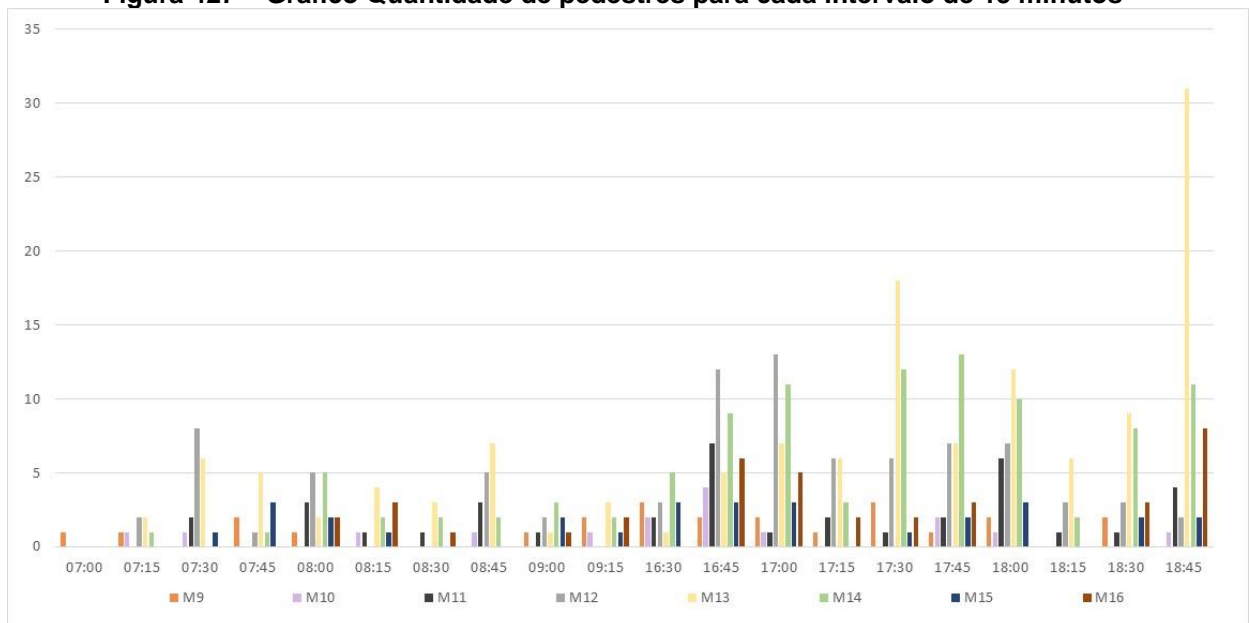
Figura 427 – Gráfico Quantidade de pedestres para cada intervalo de 15 minutos
