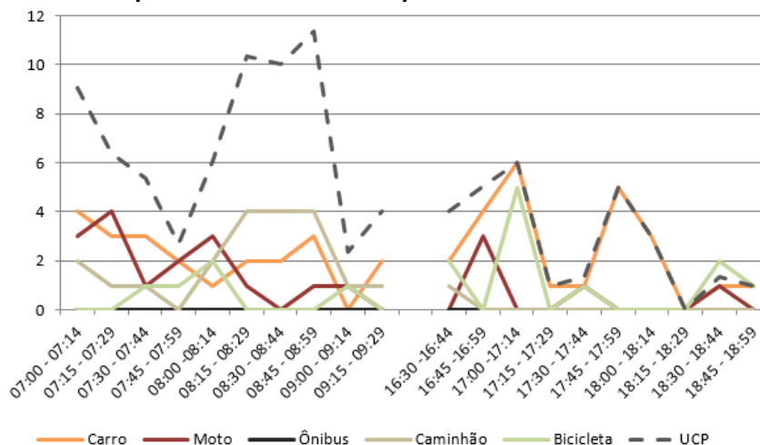
Figura 145 – Gráfico quantidade de veículos para cada intervalo de 15 minutos no M 8
