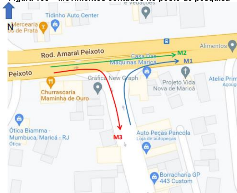
Figura 105 – Movimentos contados no posto de pesquisa
