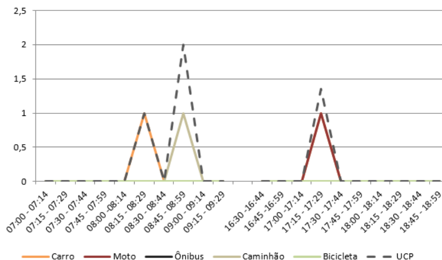
Figura 151 – Gráfico quantidade de veículos para cada intervalo de 15 minutos no M 4
