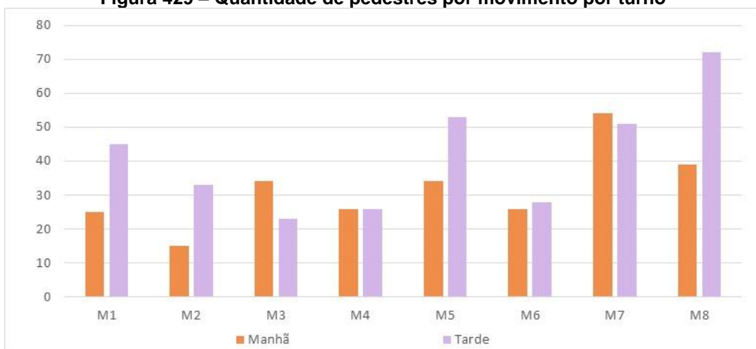
Figura 429 – Quantidade de pedestres por movimento por turno
