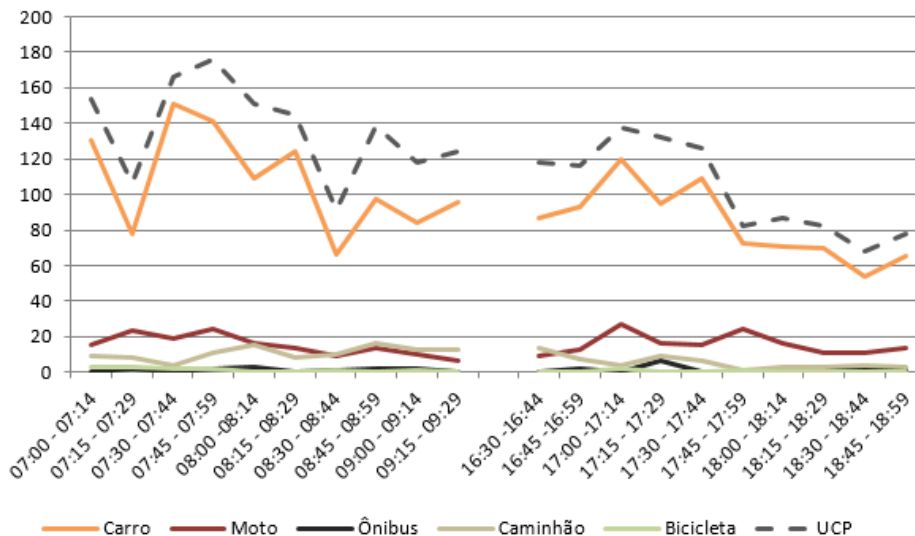
Figura 136 – Gráfico quantidade de veículos para cada intervalo de 15 minutos no M 10
