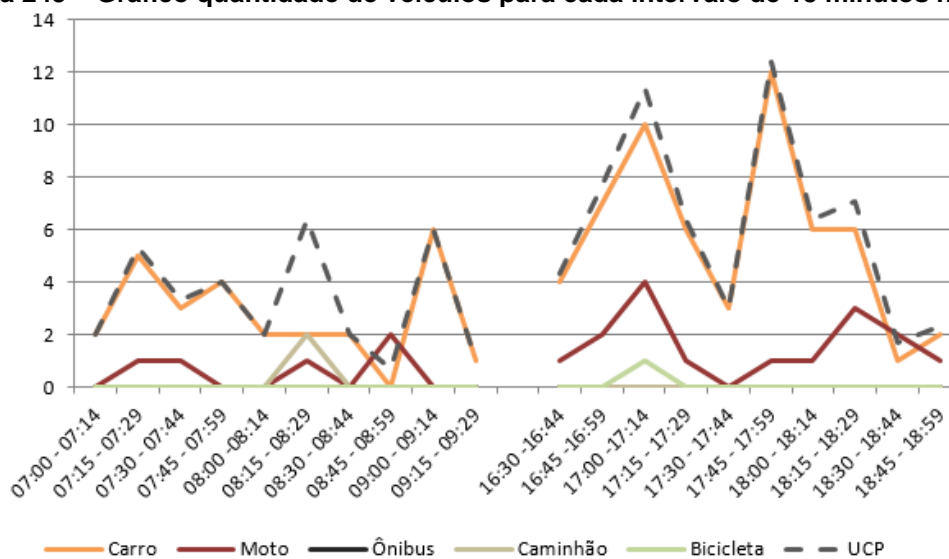
Figura 245 – Gráfico quantidade de veículos para cada intervalo de 15 minutos no M 11
