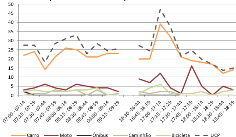
Figura 242 – Gráfico quantidade de veículos para cada intervalo de 15 minutos no M 8
