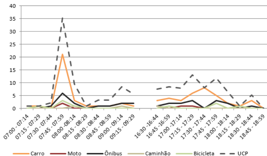
Figura 92 – Gráfico quantidade de veículos para cada intervalo de 15 minutos no M 11
