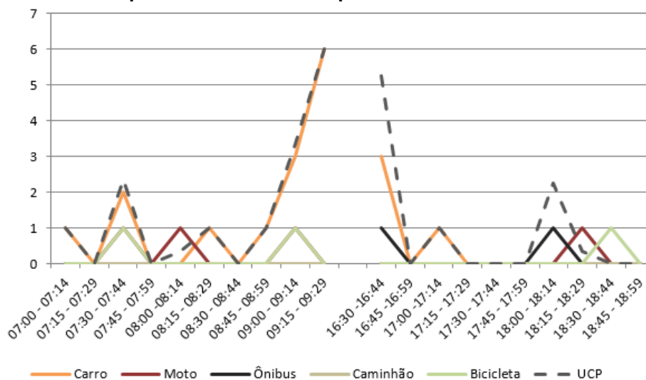
Figura 206 – Gráfico quantidade de veículos para cada intervalo de 15 minutos no M 7
