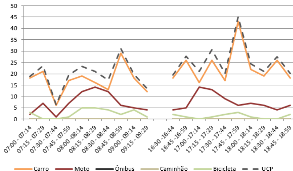
Figura 175 – Gráfico quantidade de veículos para cada intervalo de 15 minutos no M 8
