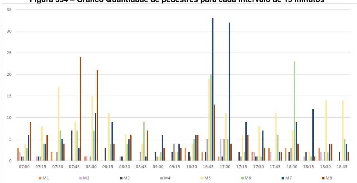
Figura 354 – Gráfico Quantidade de pedestres para cada intervalo de 15 minutos
