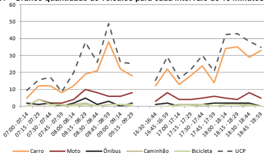
Figura 224 – Gráfico quantidade de veículos para cada intervalo de 15 minutos no M 8
