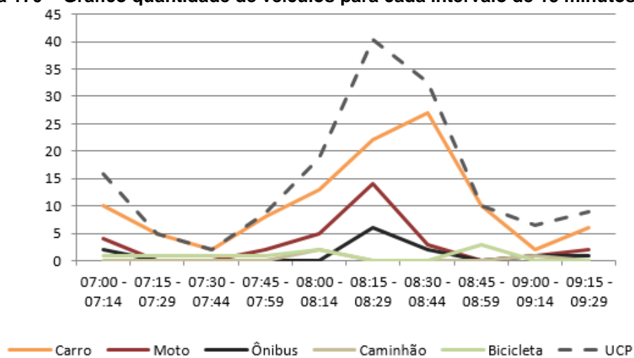
Figura 170 – Gráfico quantidade de veículos para cada intervalo de 15 minutos no M 3
