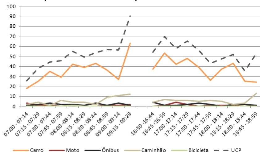
Figura 139 – Gráfico quantidade de veículos para cada intervalo de 15 minutos no M 1
