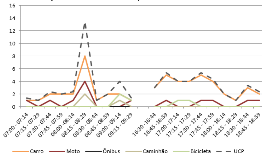
Figura 152 – Gráfico quantidade de veículos para cada intervalo de 15 minutos no M 5
