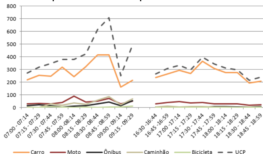
Figura 107 – Gráfico quantidade de veículos para cada intervalo de 15 minutos no M 1
