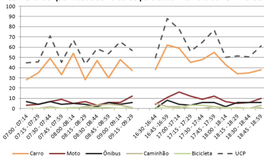
Figura 235 – Gráfico quantidade de veículos para cada intervalo de 15 minutos no M 1
