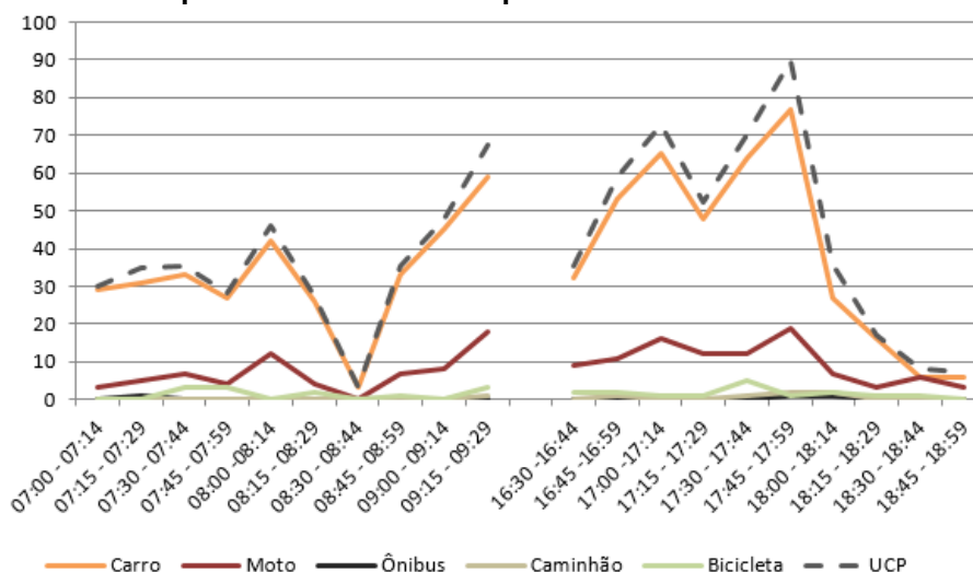
Figura 116 – Gráfico quantidade de veículos para cada intervalo de 15 minutos no M 5
