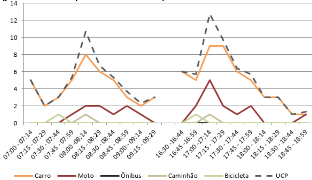
Figura 197 – Gráfico quantidade de veículos para cada intervalo de 15 minutos no M 13
