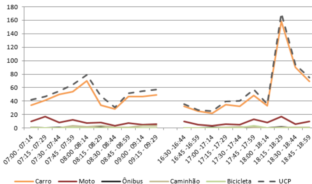
Figura 213 – Gráfico quantidade de veículos para cada intervalo de 15 minutos no M 4
