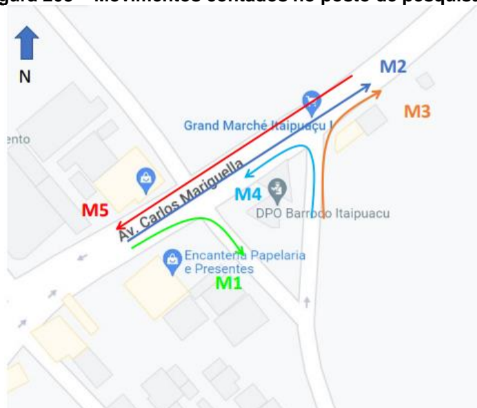
Figura 208 – Movimentos contados no posto de pesquisa 15
