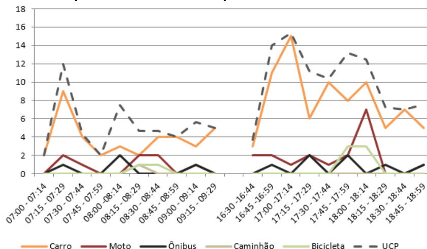
Figura 89 – Gráfico quantidade de veículos para cada intervalo de 15 minutos no M 8
