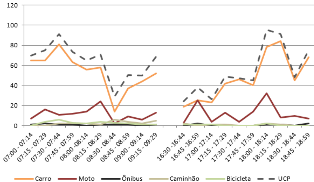
Figura 214 – Gráfico quantidade de veículos para cada intervalo de 15 minutos no M 5
